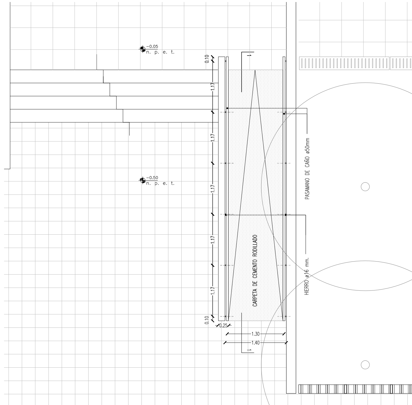
CORTE 1-1 ESC. 1:50
