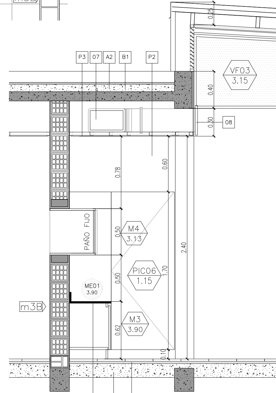
CORTE B-B
