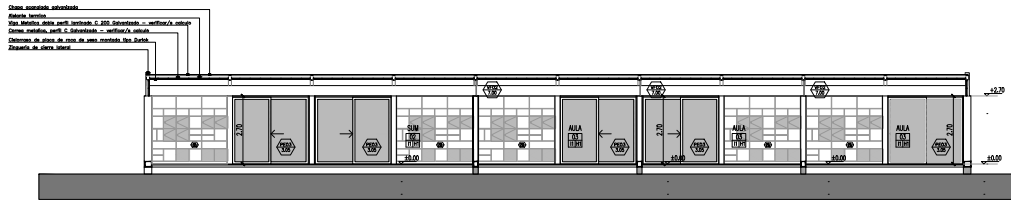
CORTE 3
