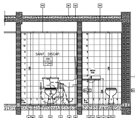
CORTE D-D
