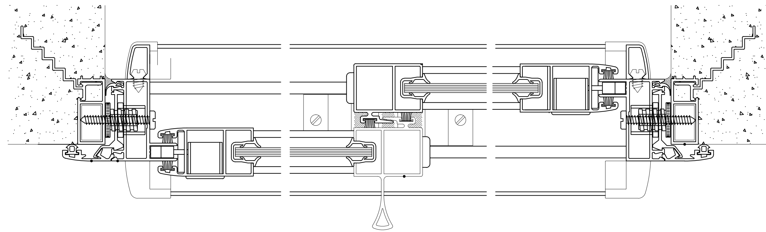
DETALLE DE VENTANAS - CORTE HORIZONTAL 1:5
