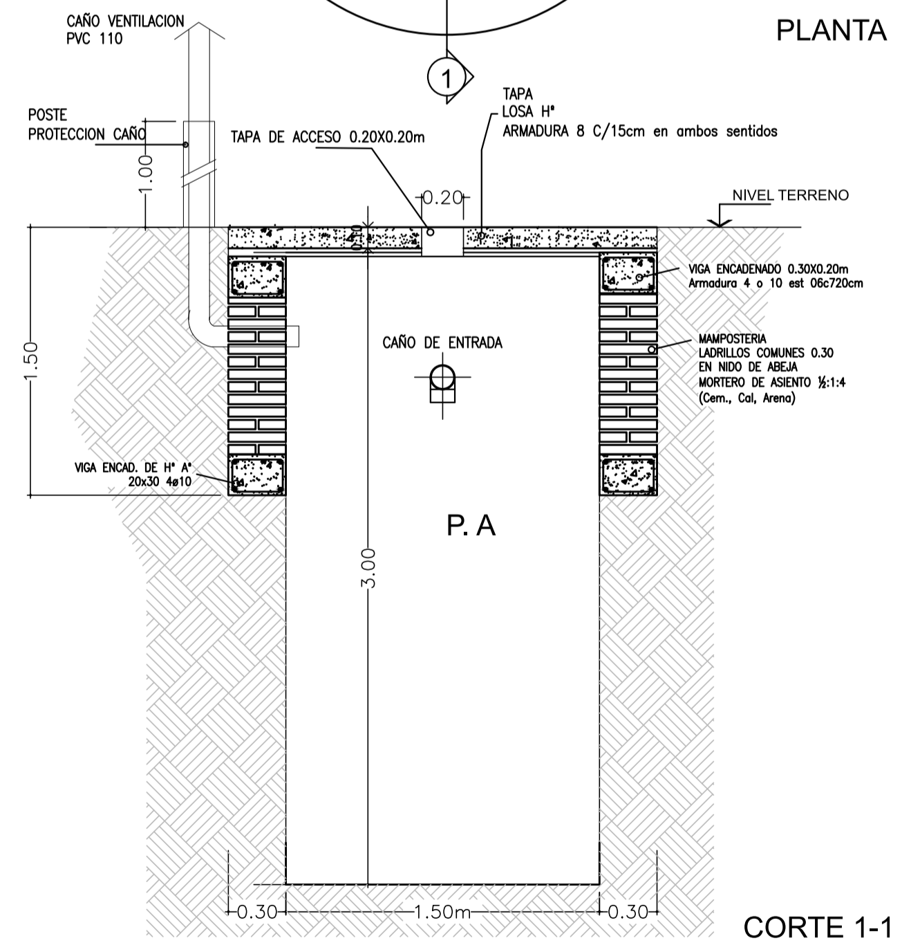
DETALLE POZO ABSORBENTE Esc 1:25
