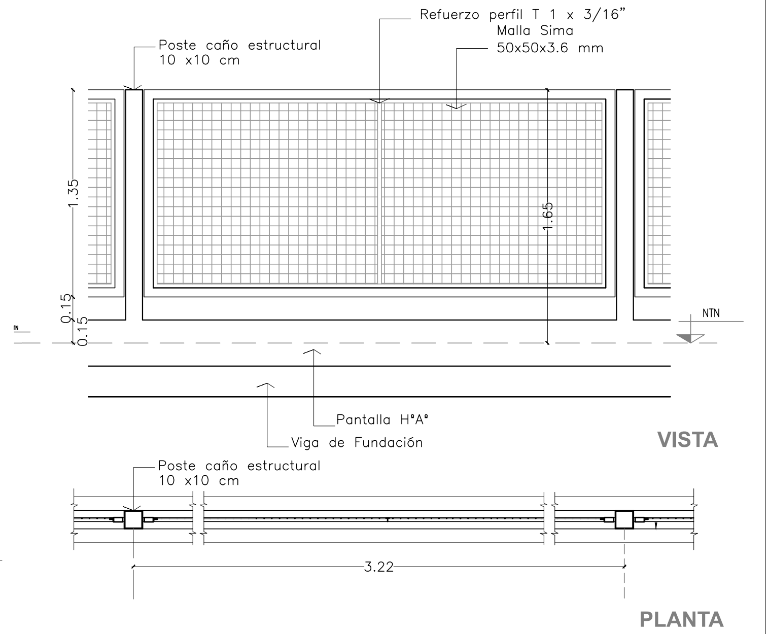
DETALLE CERCO MALLA SIMA - Esc 1/25
