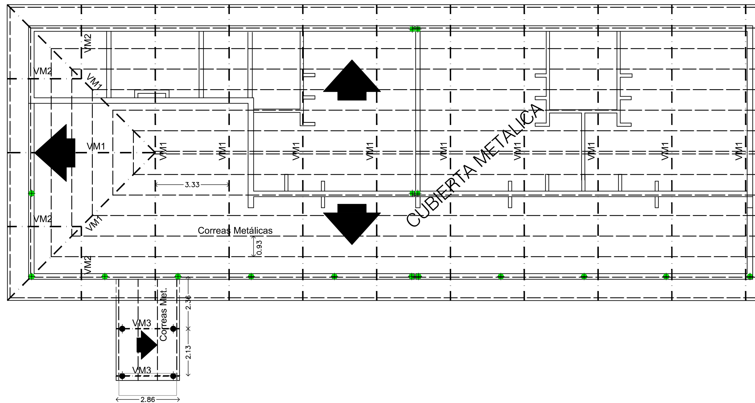
PLANTA ESTR. DE TECHOS
