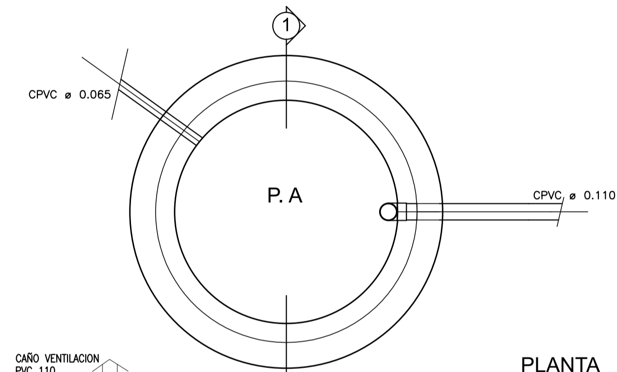
PLANTA
