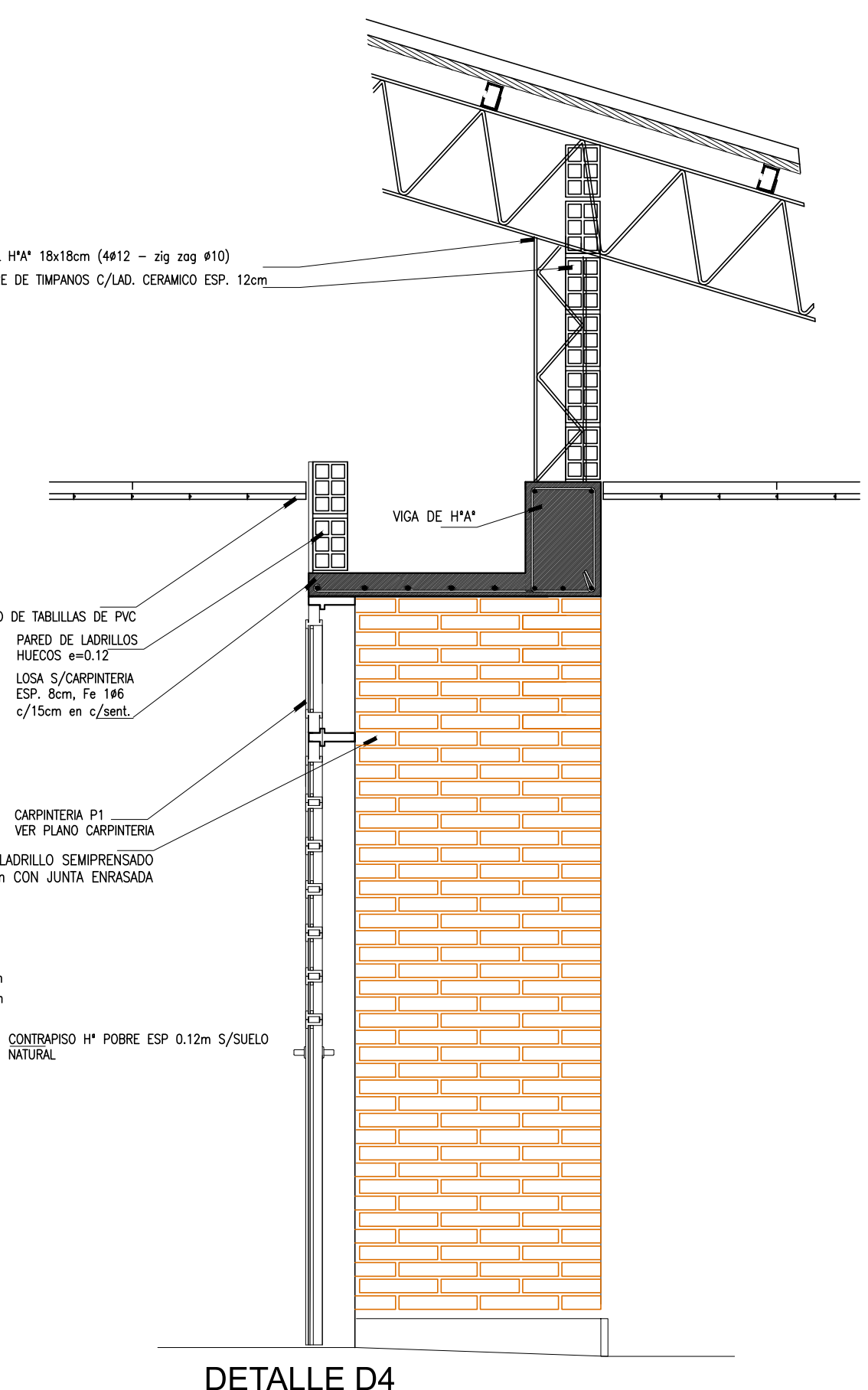
DETALLE D4
