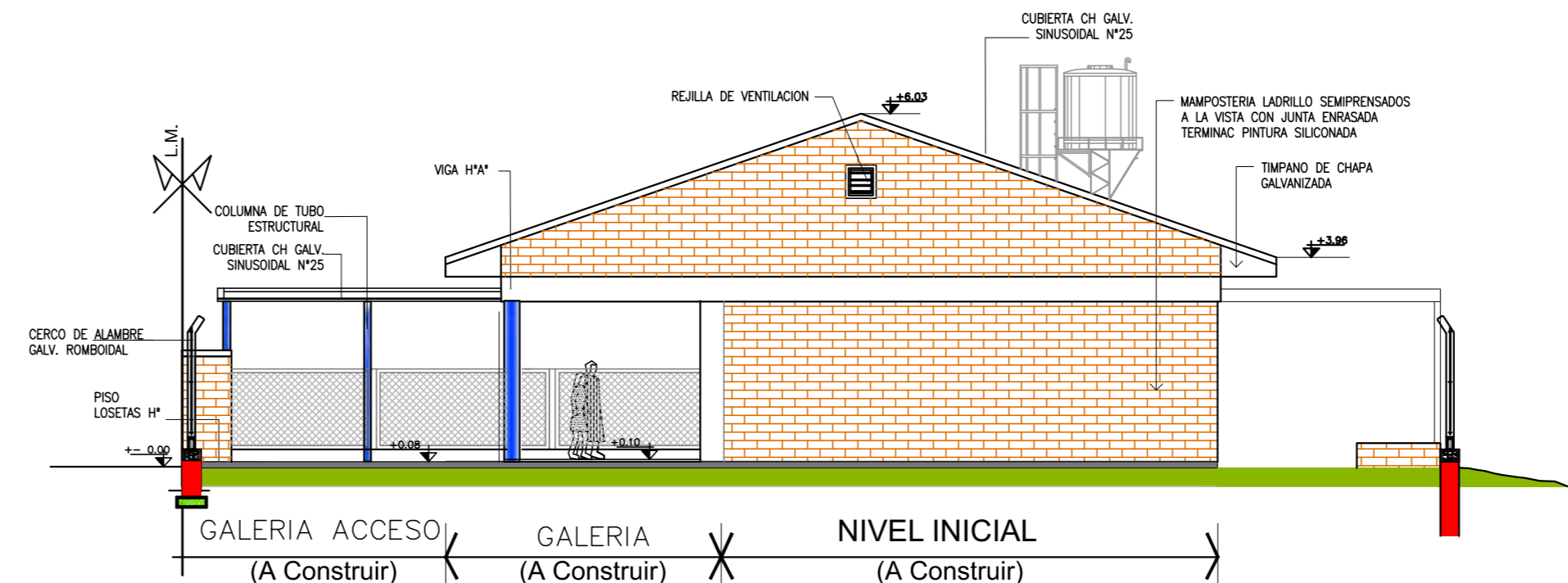
VISTA LATERAL Esc 1:100
