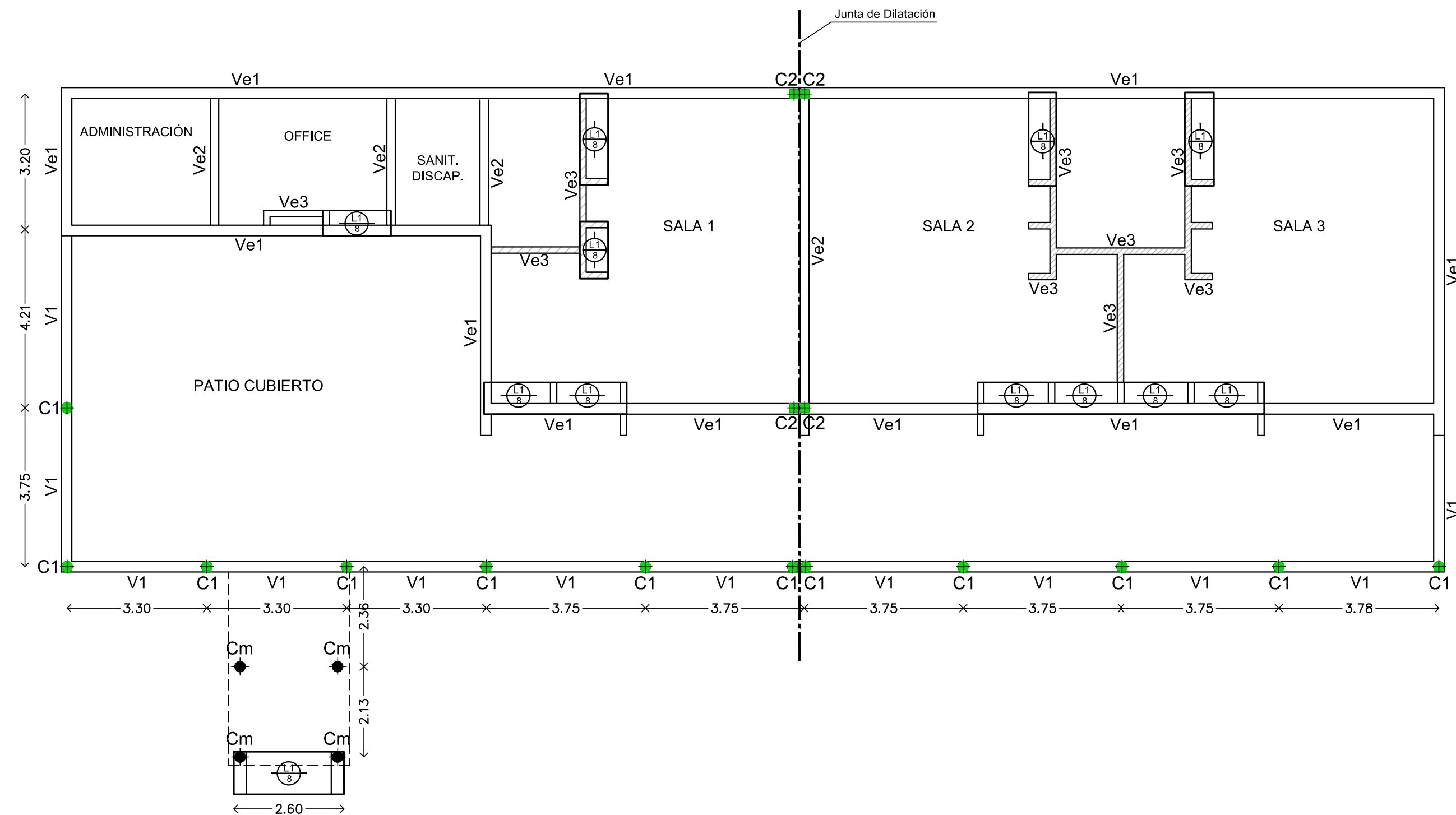
PLANTA ESTRUCTURAS +3.00m
