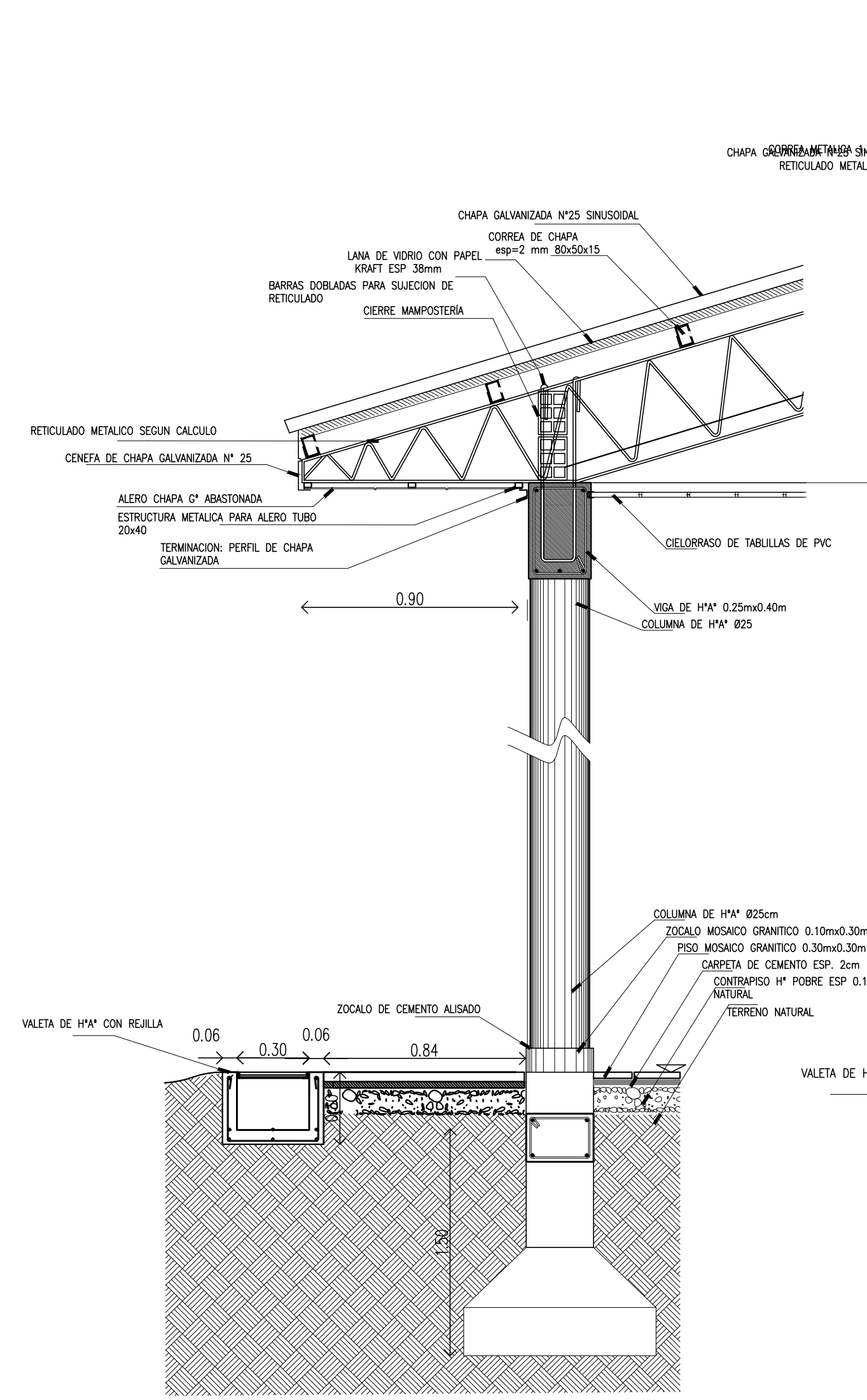
DETALLE D2
