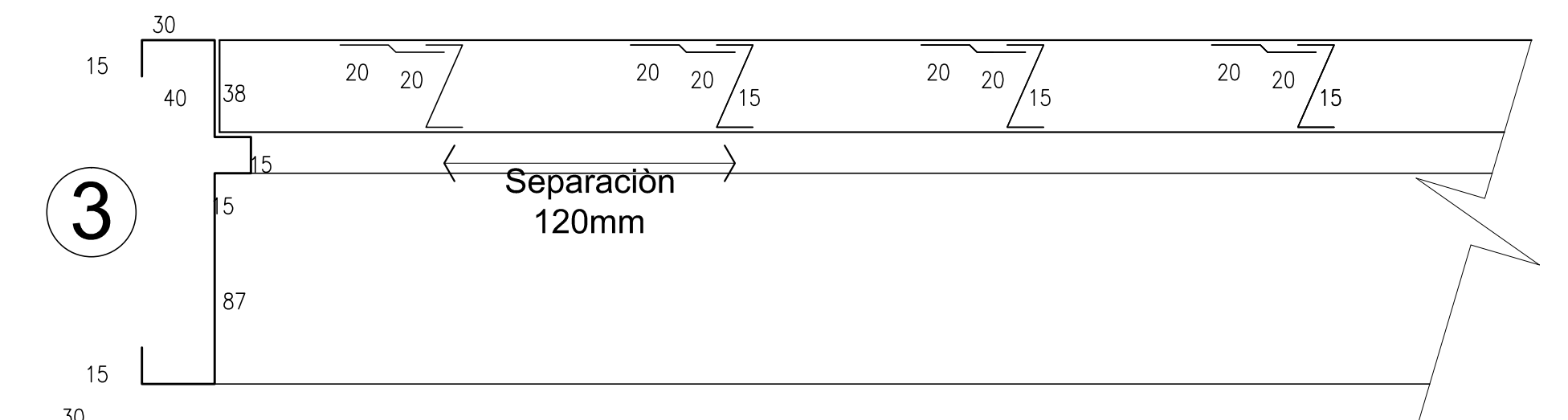
DETALLE DE PUERTAS - CORTE HORIZONTAL 1:5
