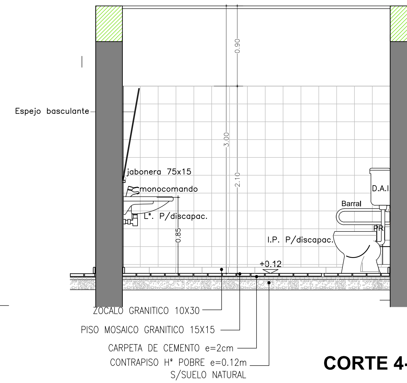
CORTE 3-3
