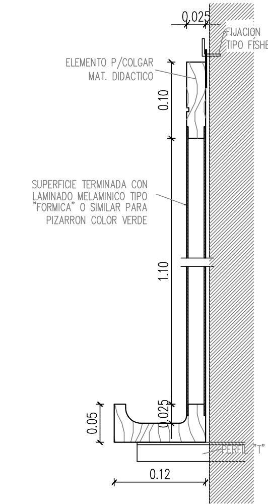
DETALLE PIZARRON Esc 1/5
