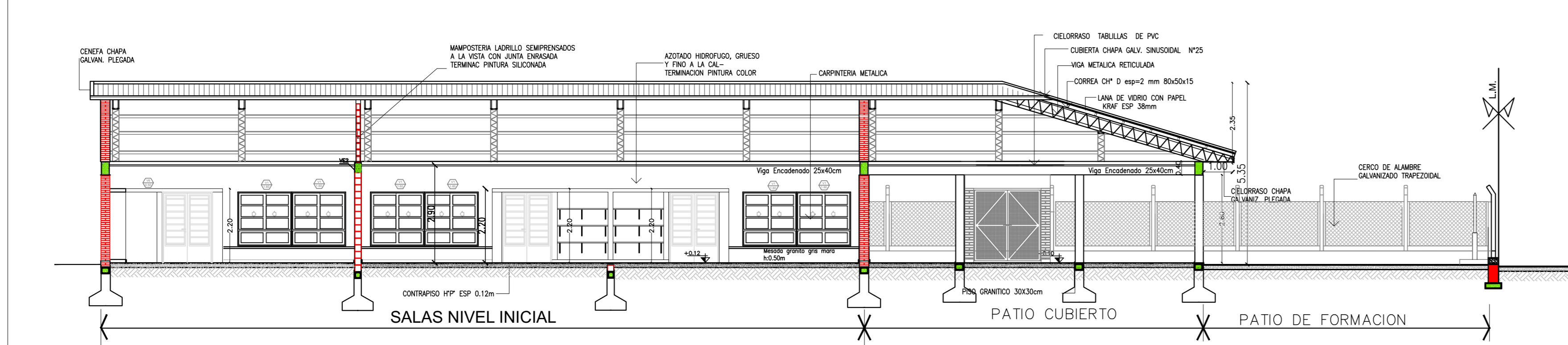
CORTE LONGITUDINAL "A-A" Esc 1:100
