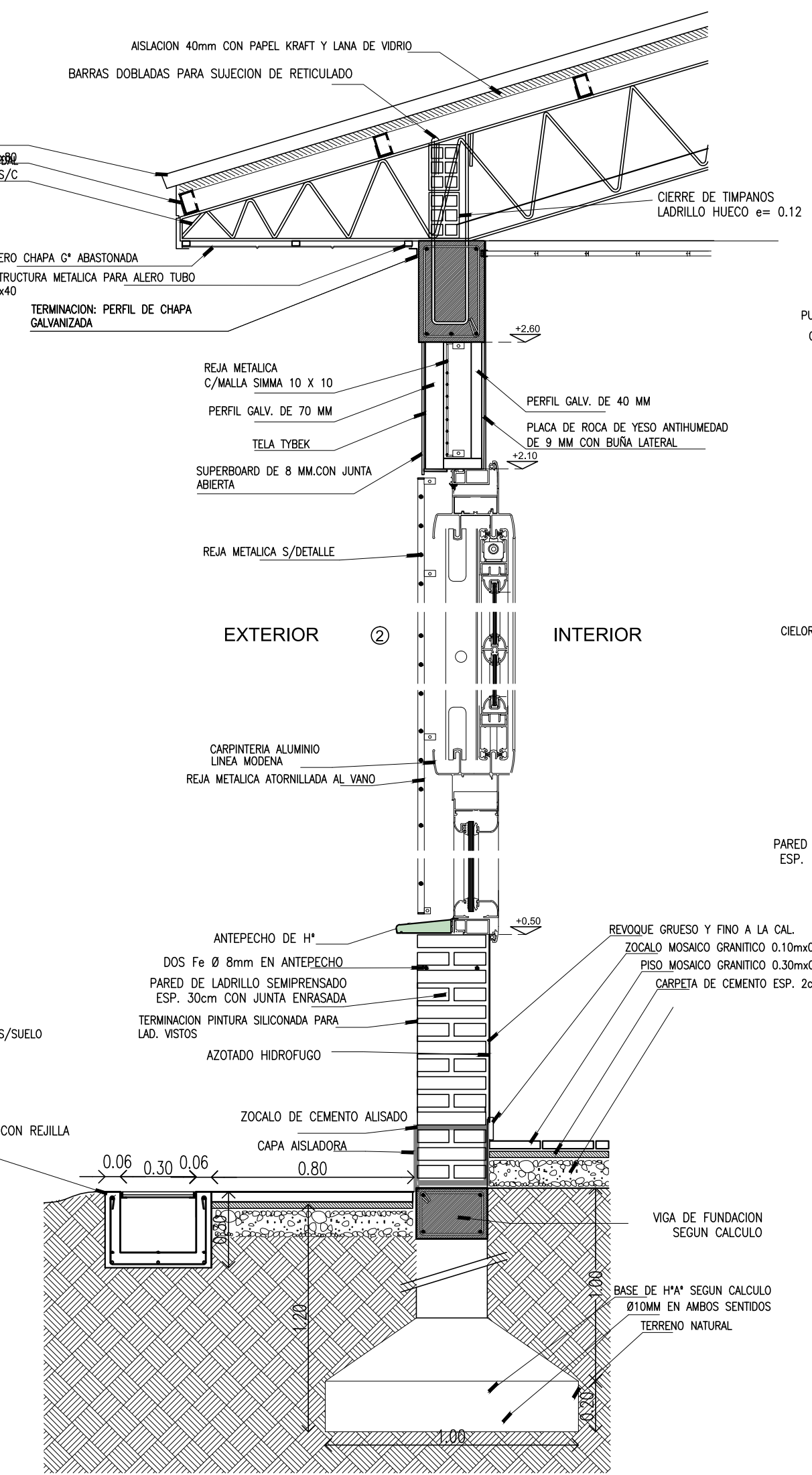
DETALLE D3
