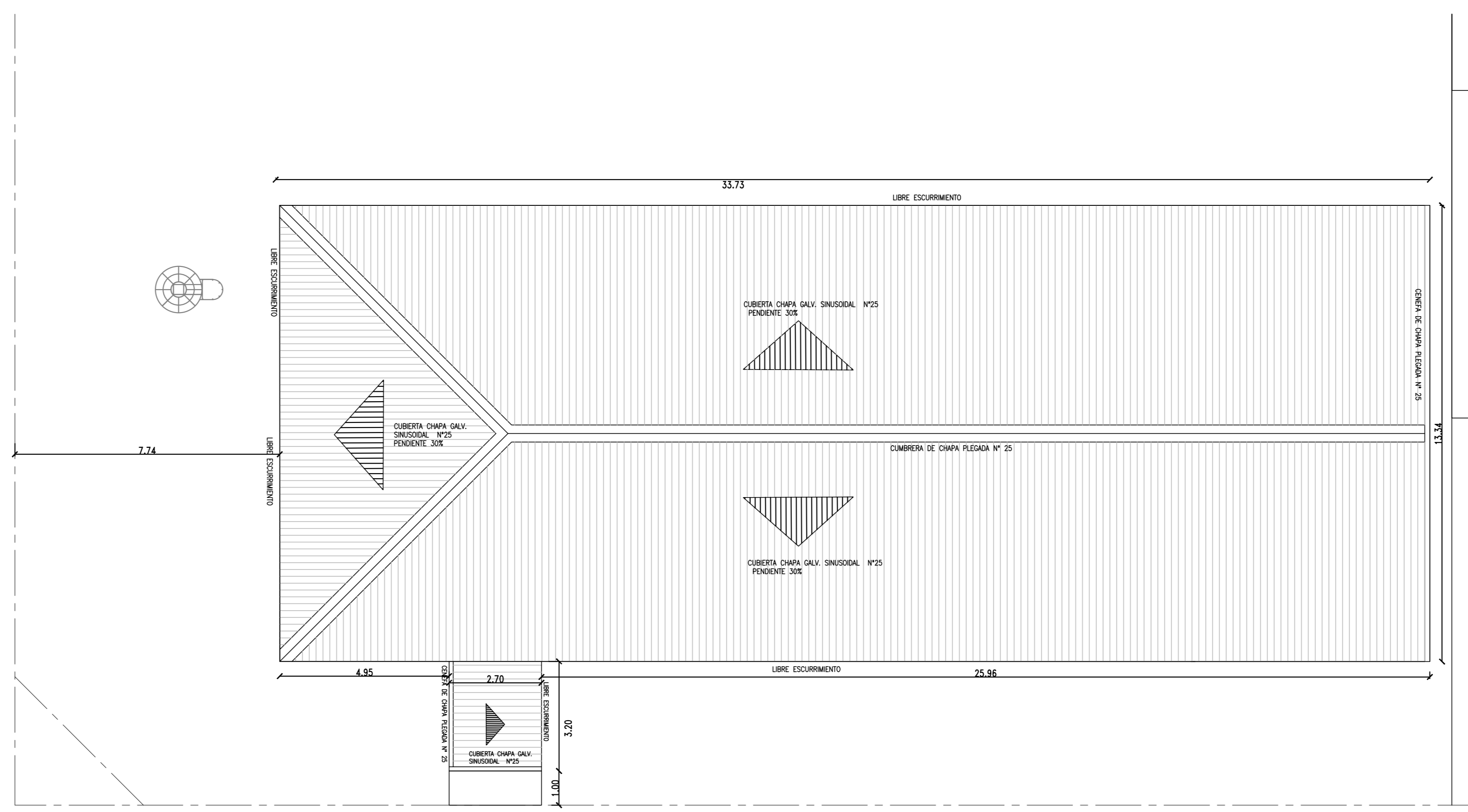
PLANTA DE TECHOS Esc 1:100
