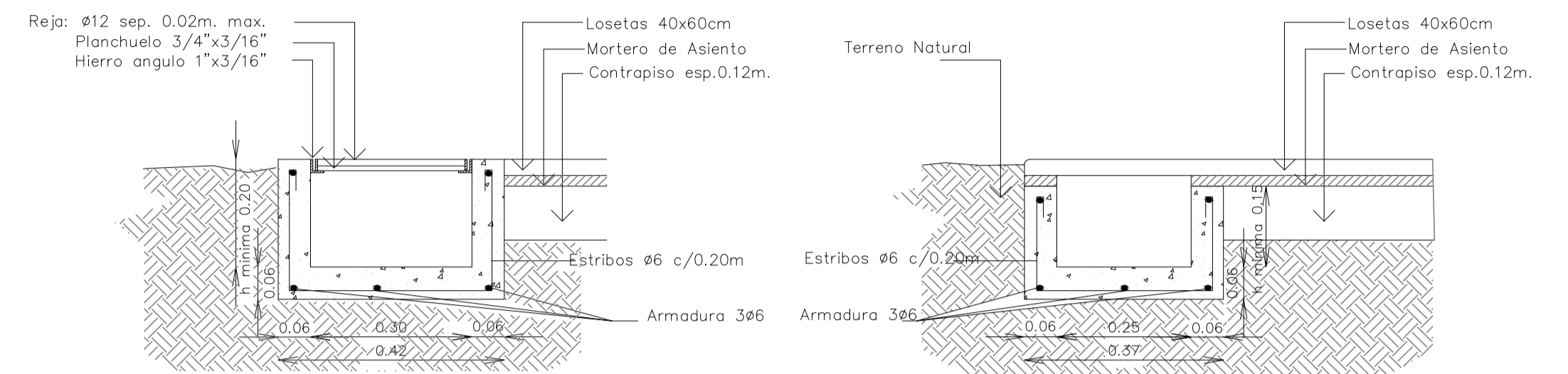
DETALLE VALETAS Esc 1:10
