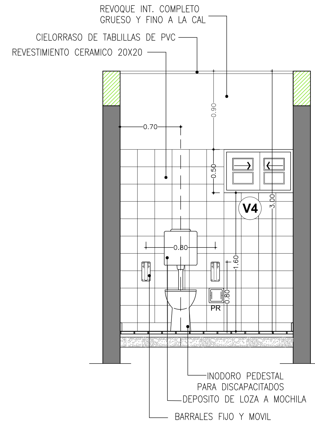
CORTE 1-1
