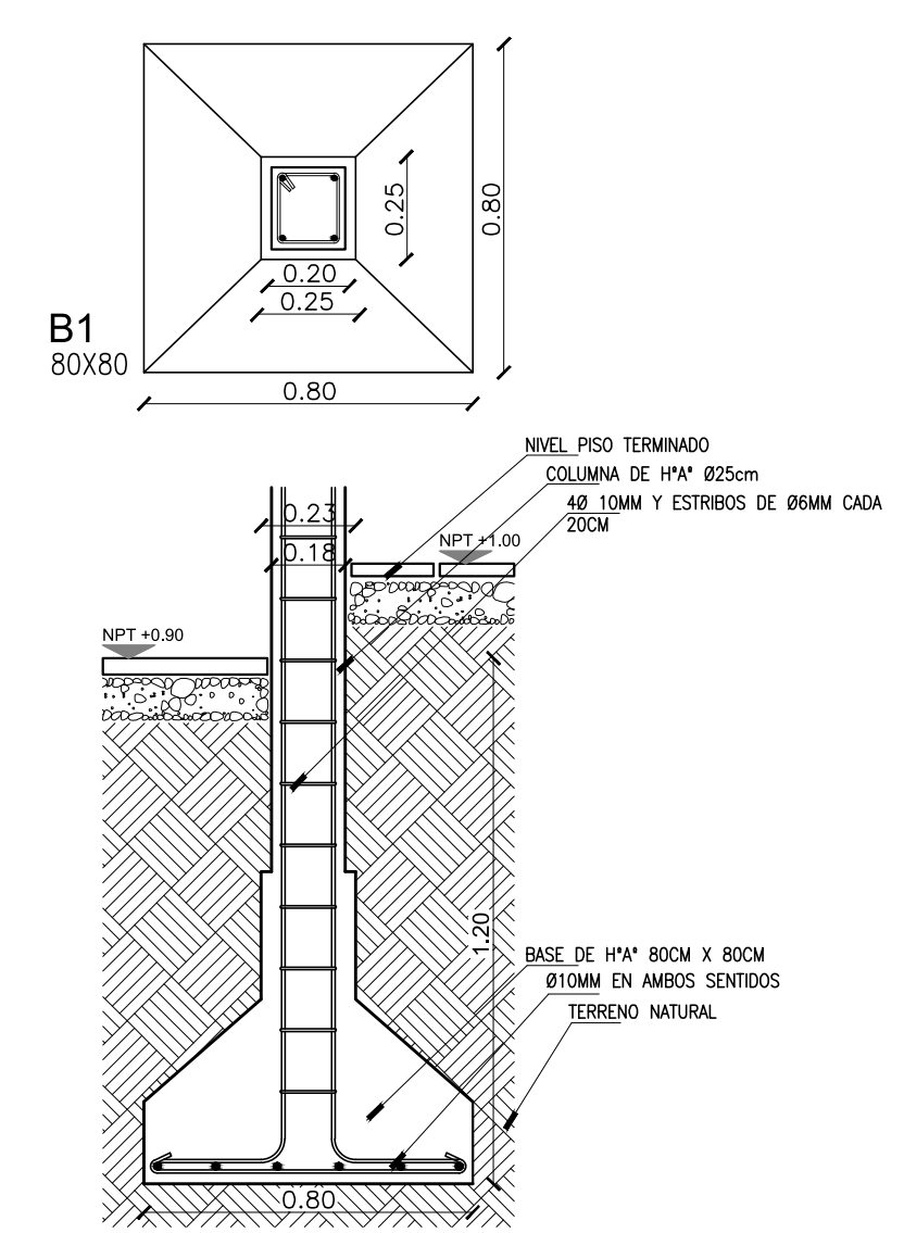
DETALLE D1
