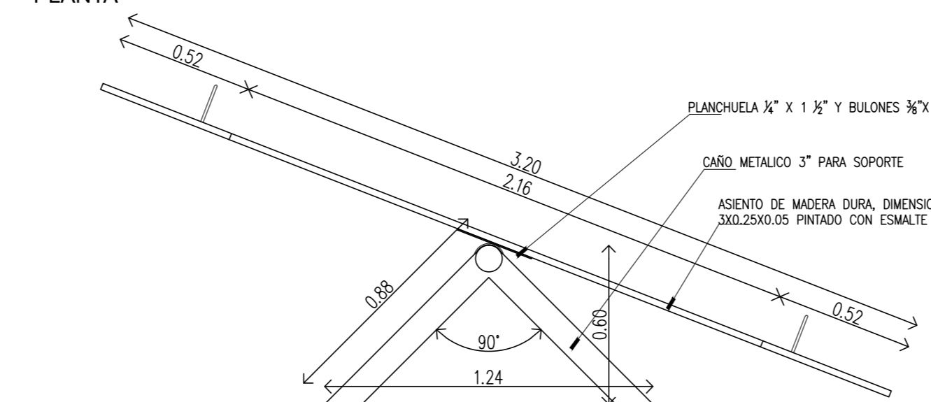
VISTA
