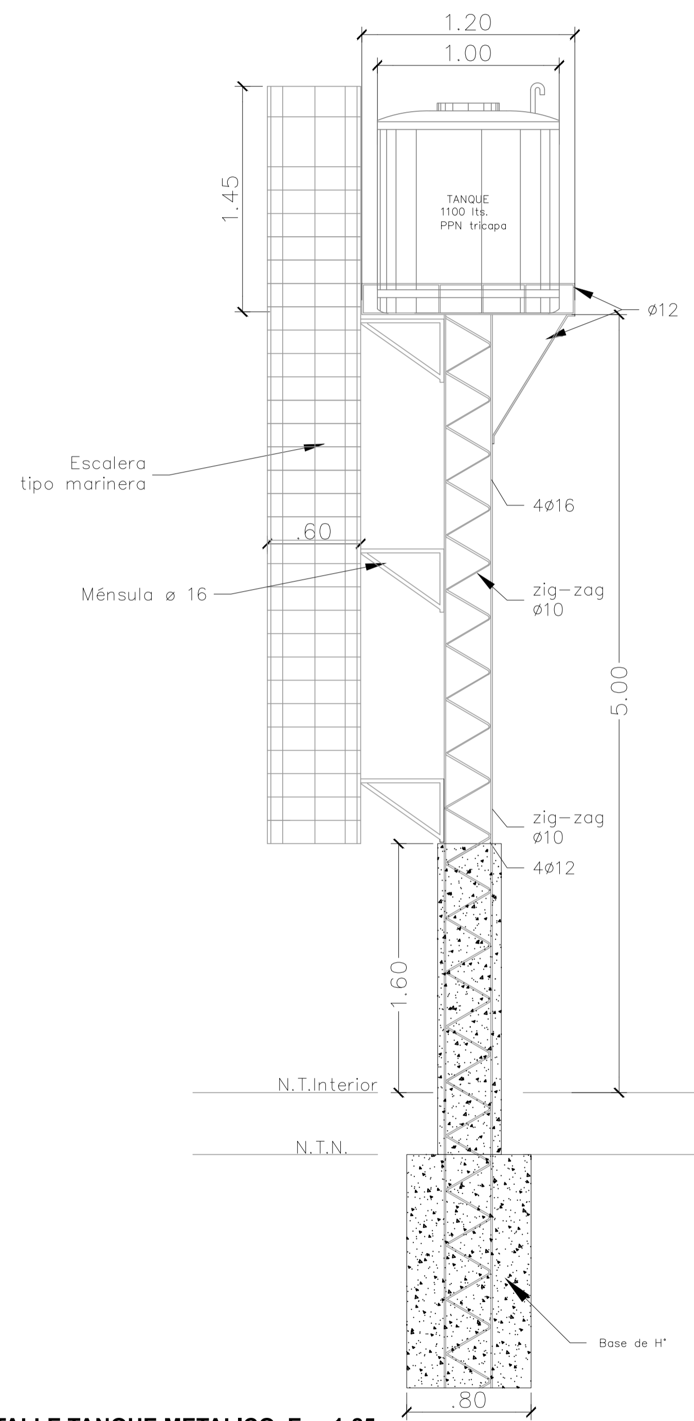
DETALLE TANQUE METALICO Esc 1:25
