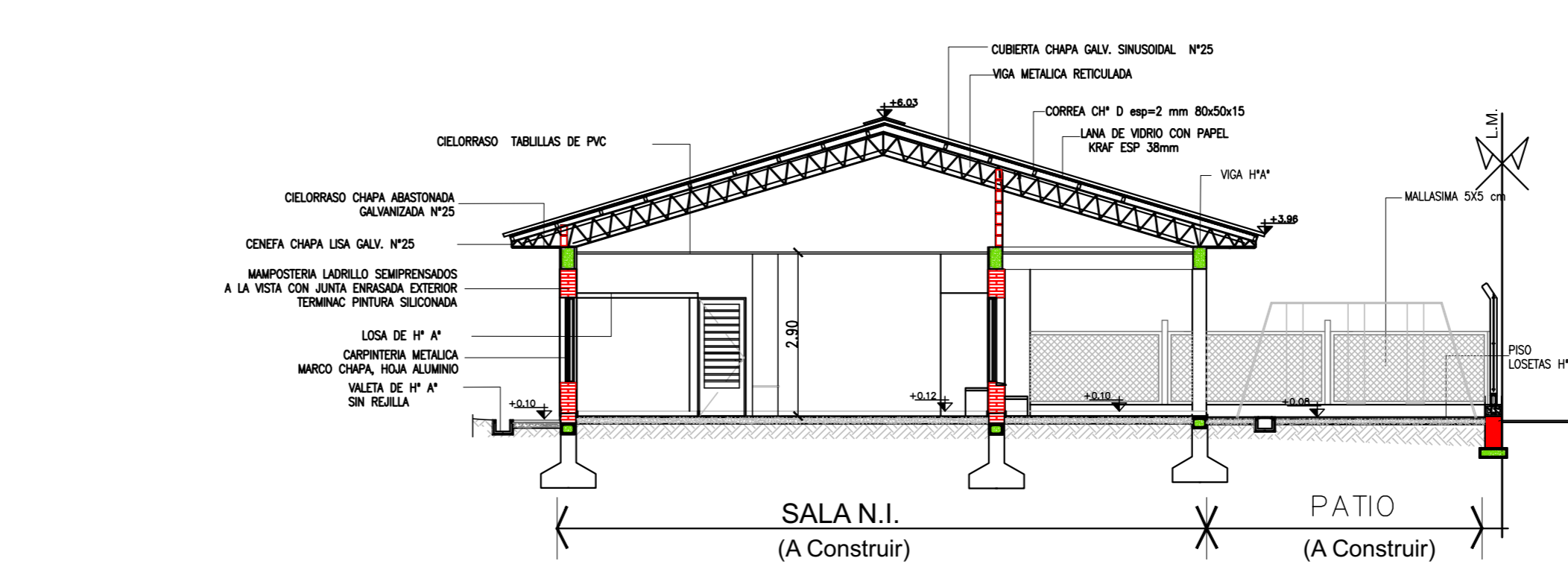
CORTE TRANSVERSAL "B-B" Esc 1:100
