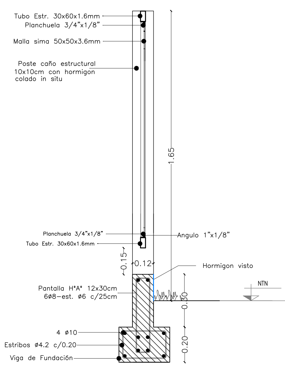
DETALLE CERCO MALLA SIMA - Esc 1/25
