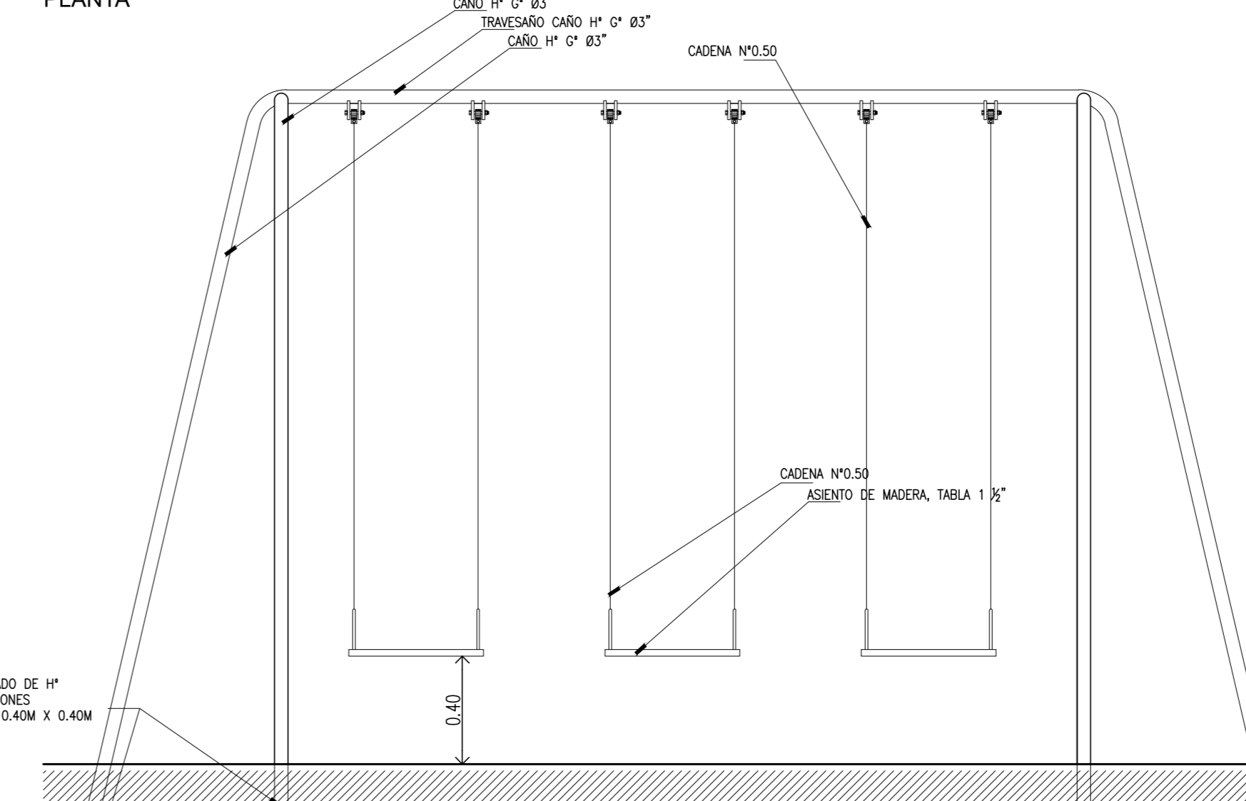
VISTA
