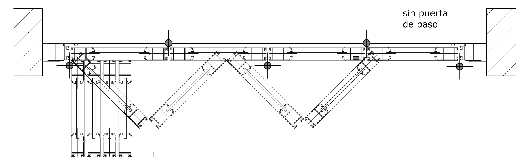
DETALLE DE PUERTAS - CORTE HORIZONTAL 1:5
