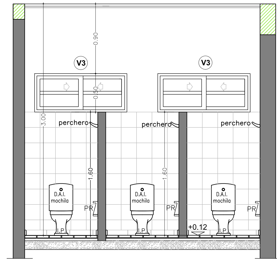
CORTE 1-1
