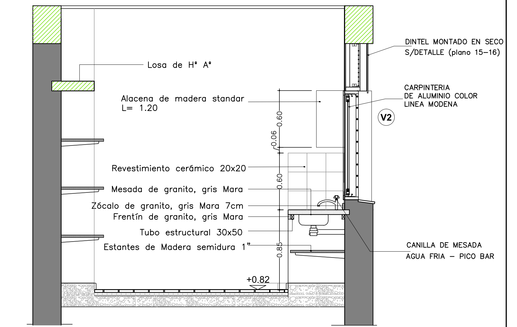
CORTE 5-5
