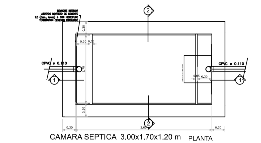
CAMARA SEPTICA 3.00x1.70x1.20 m PLANTA
