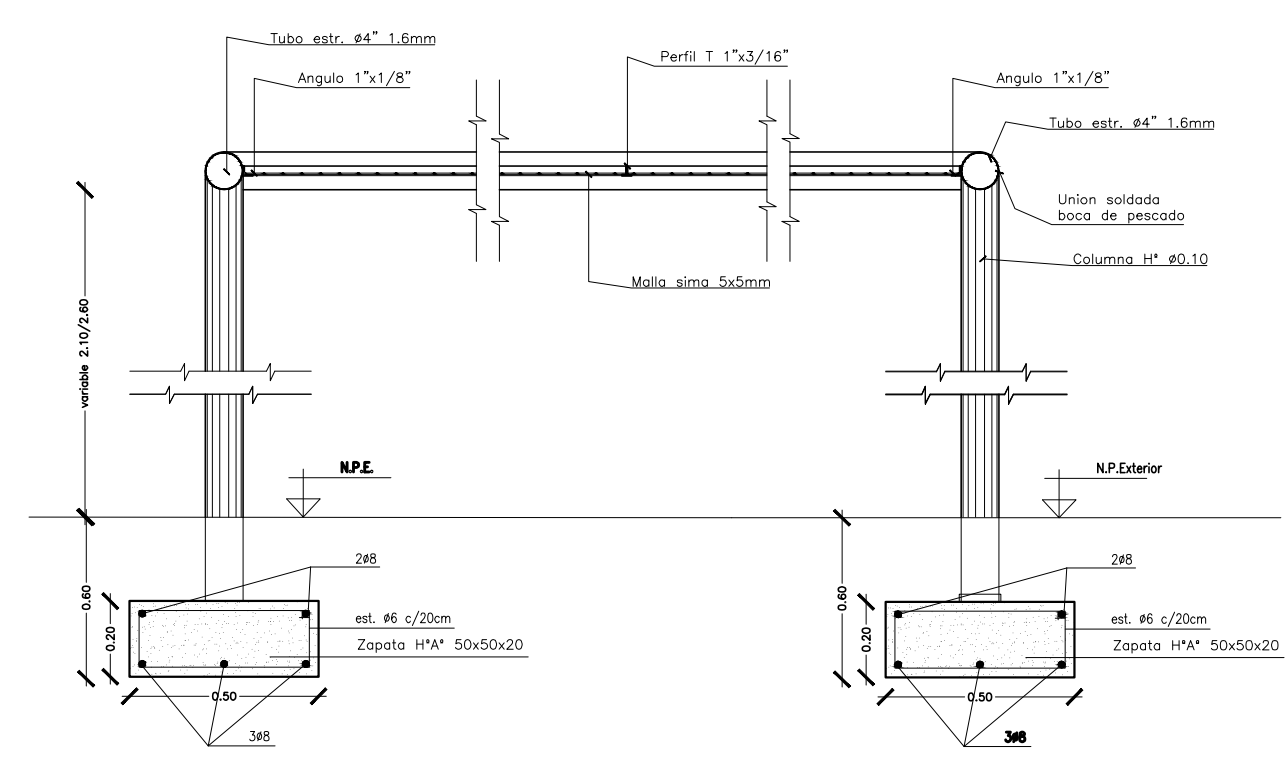
DETALLE PERGOLA Esc 1/20
