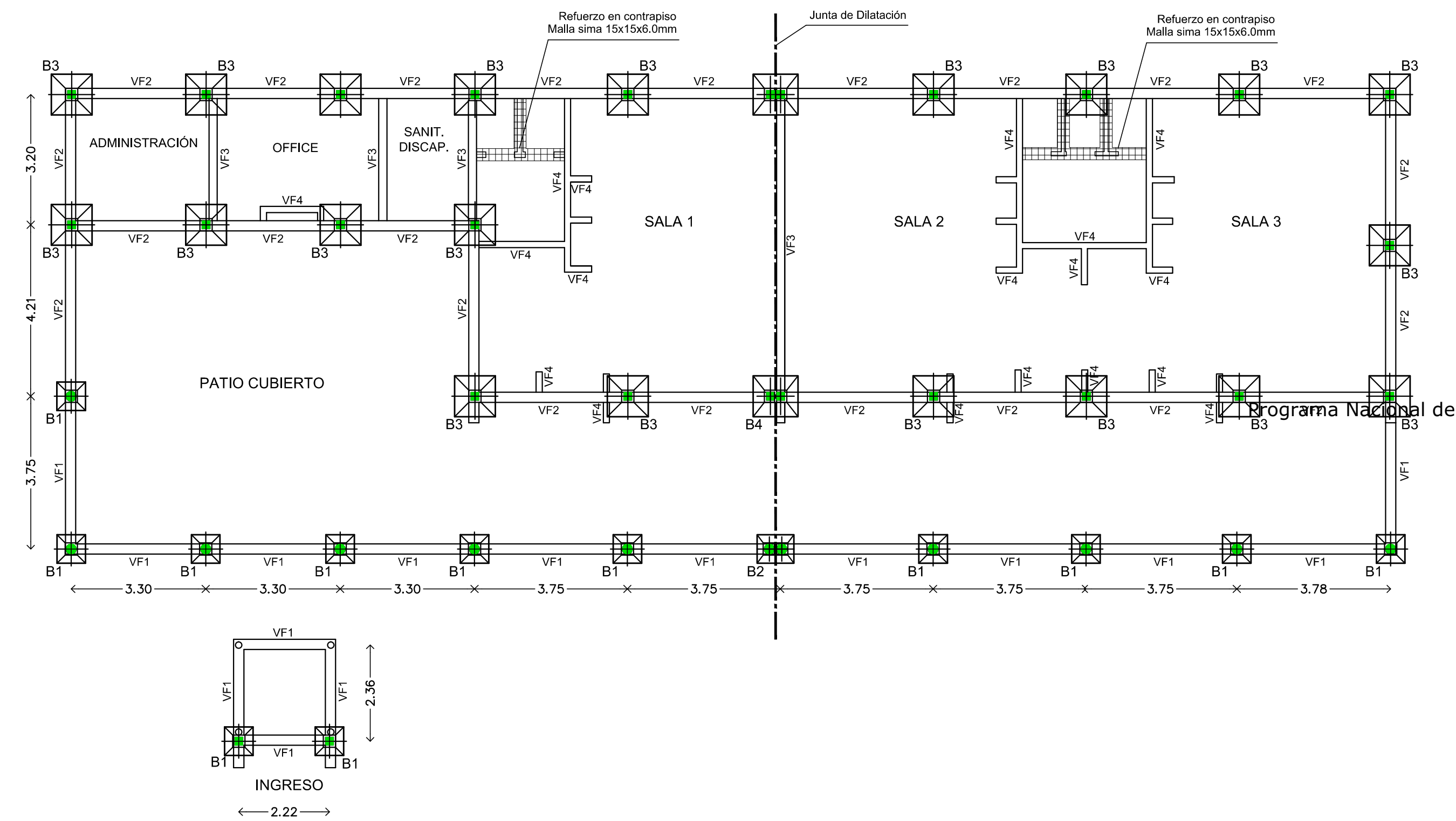
PLANTA FUNDACIONES
