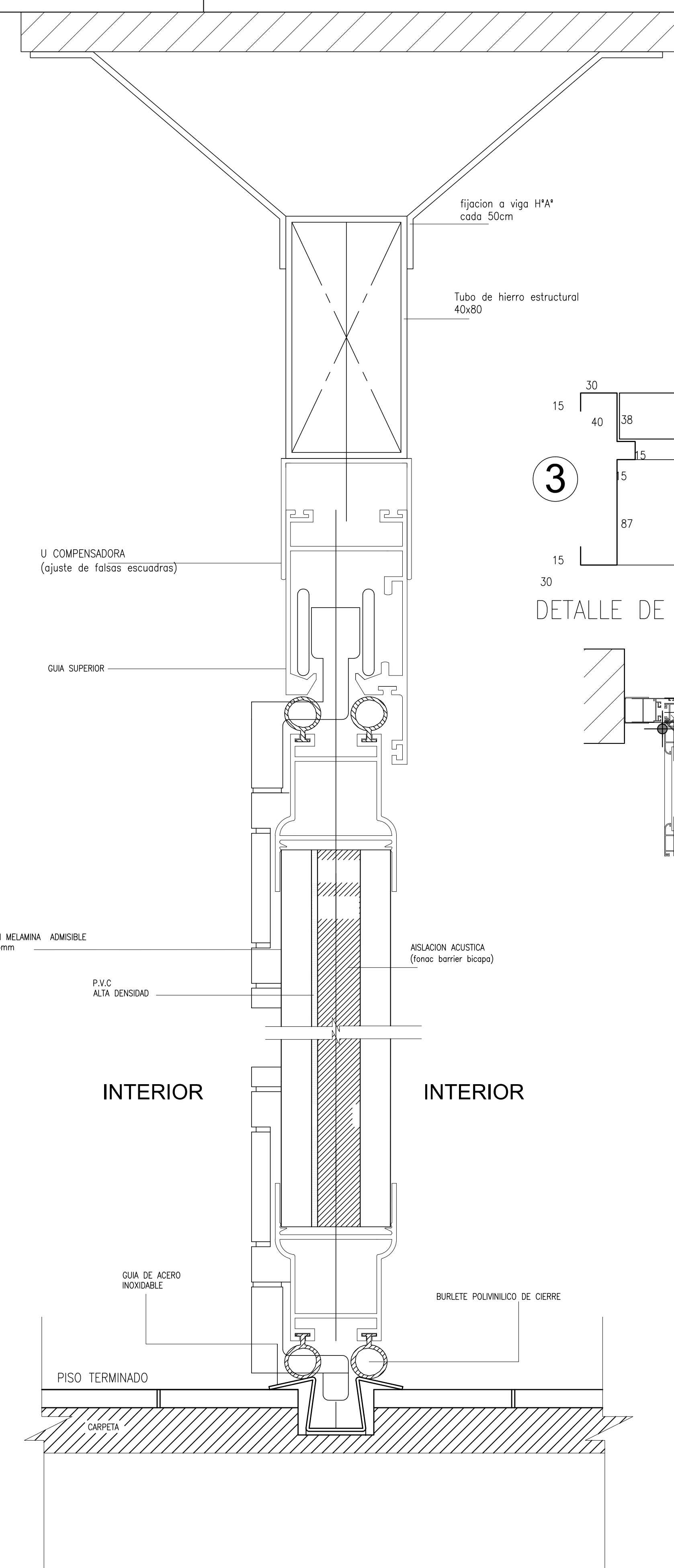
DETALLE: DIVISOR PLEGABLE CON PANEL COMPUESTO 38MM
