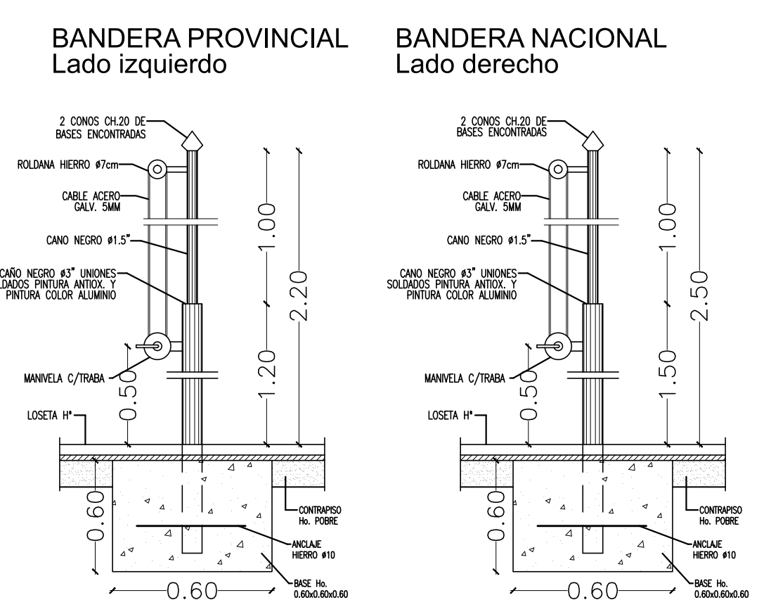
DETALLE MASTILES N.I. Esc 1/20
