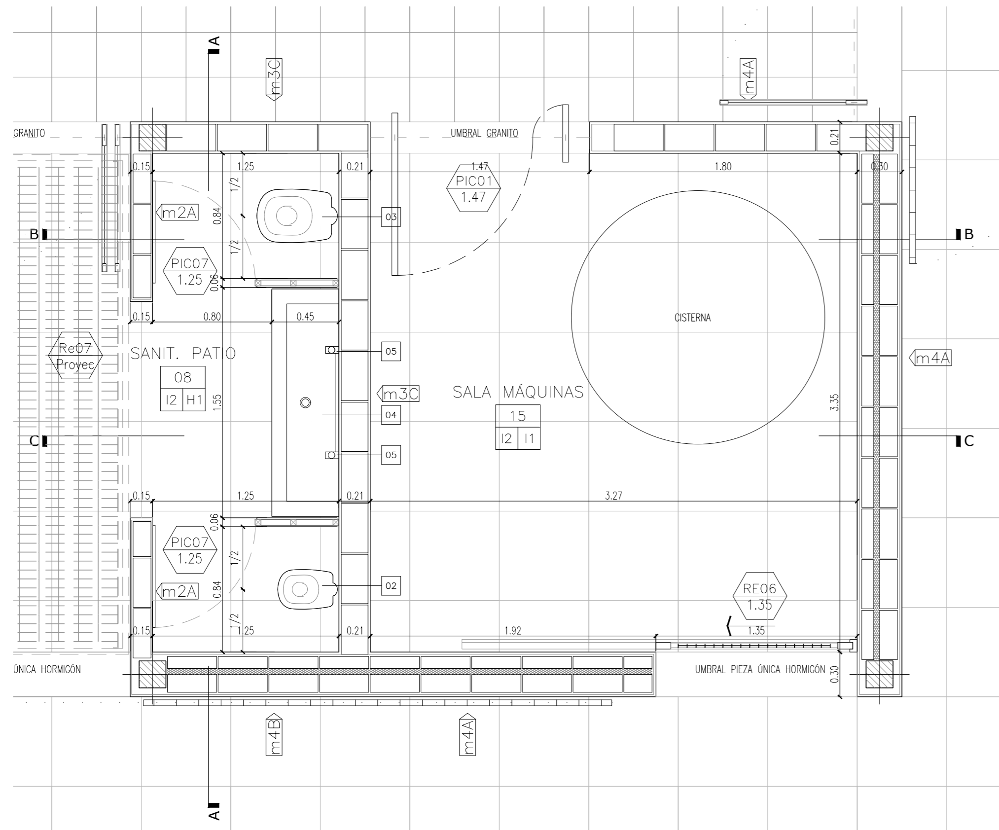
PLANTA
