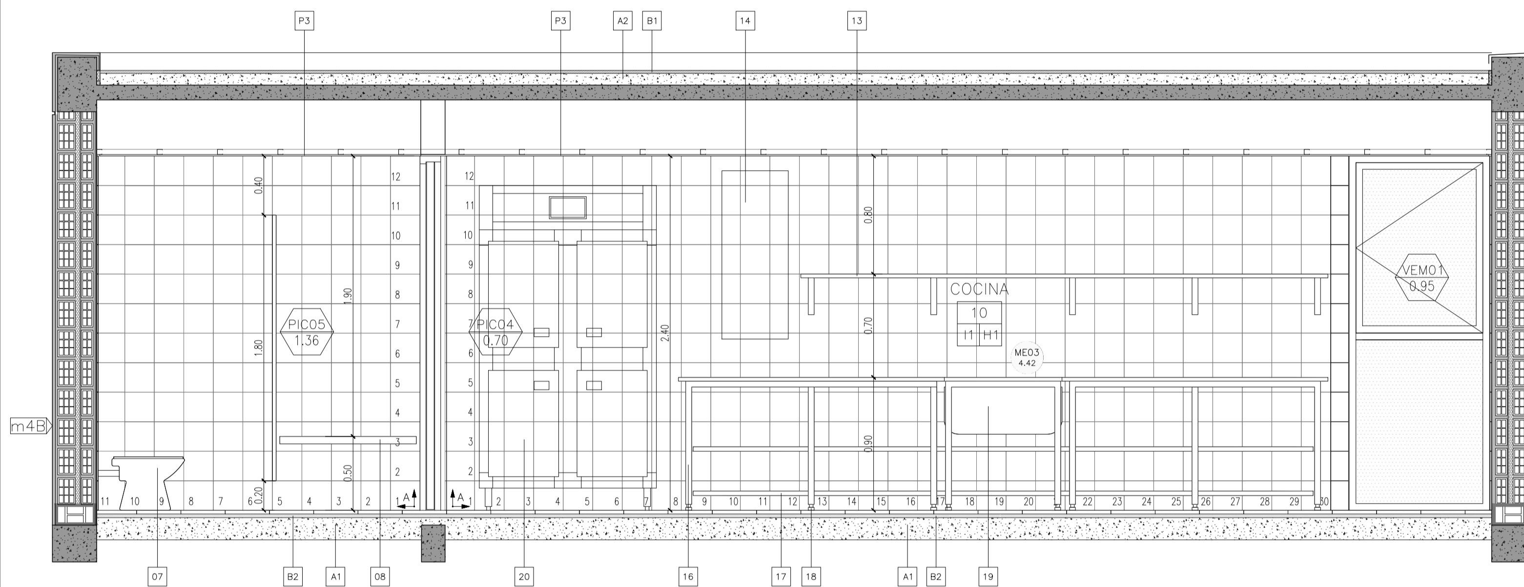
CORTE B-B
