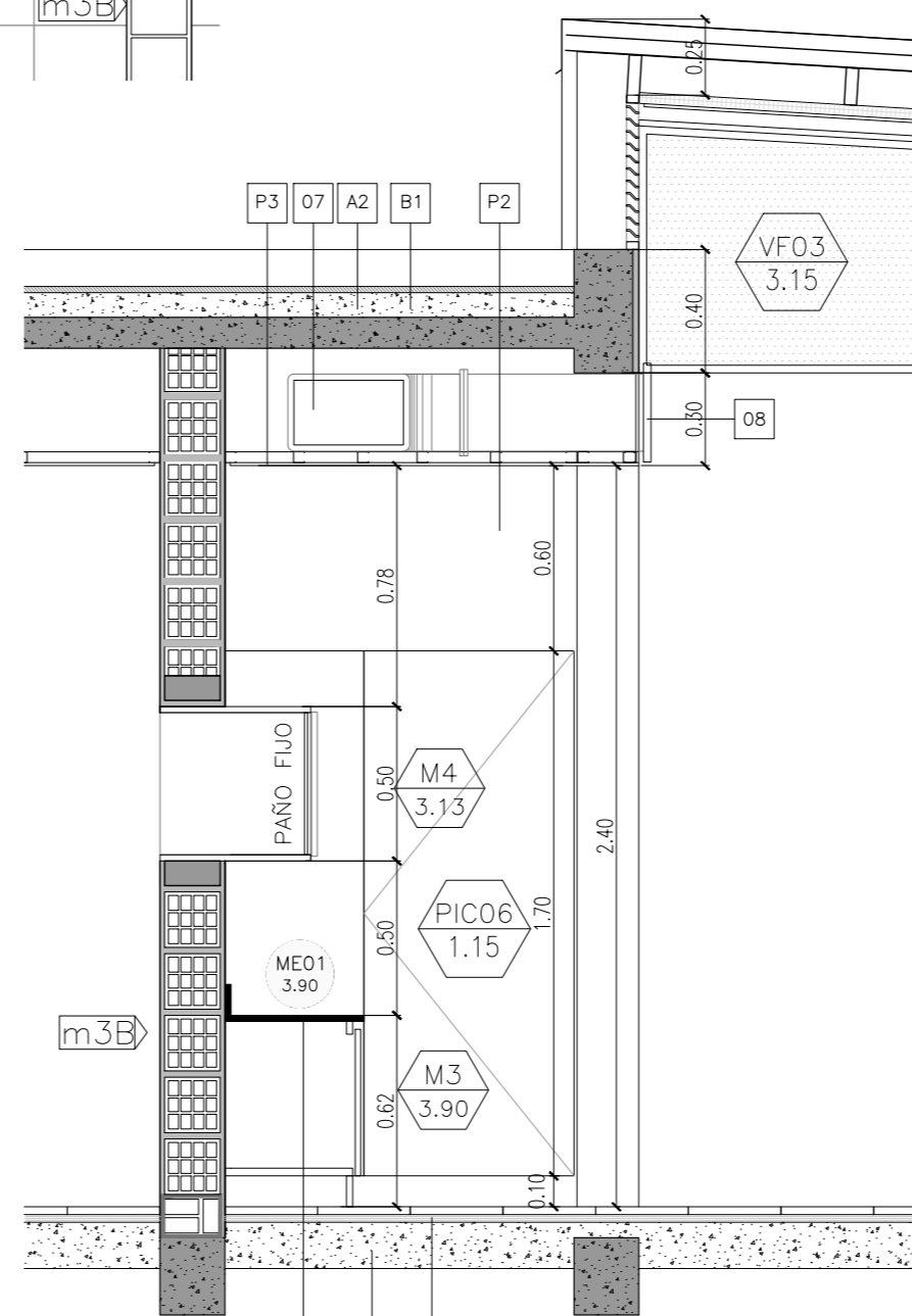
CORTE B-B
