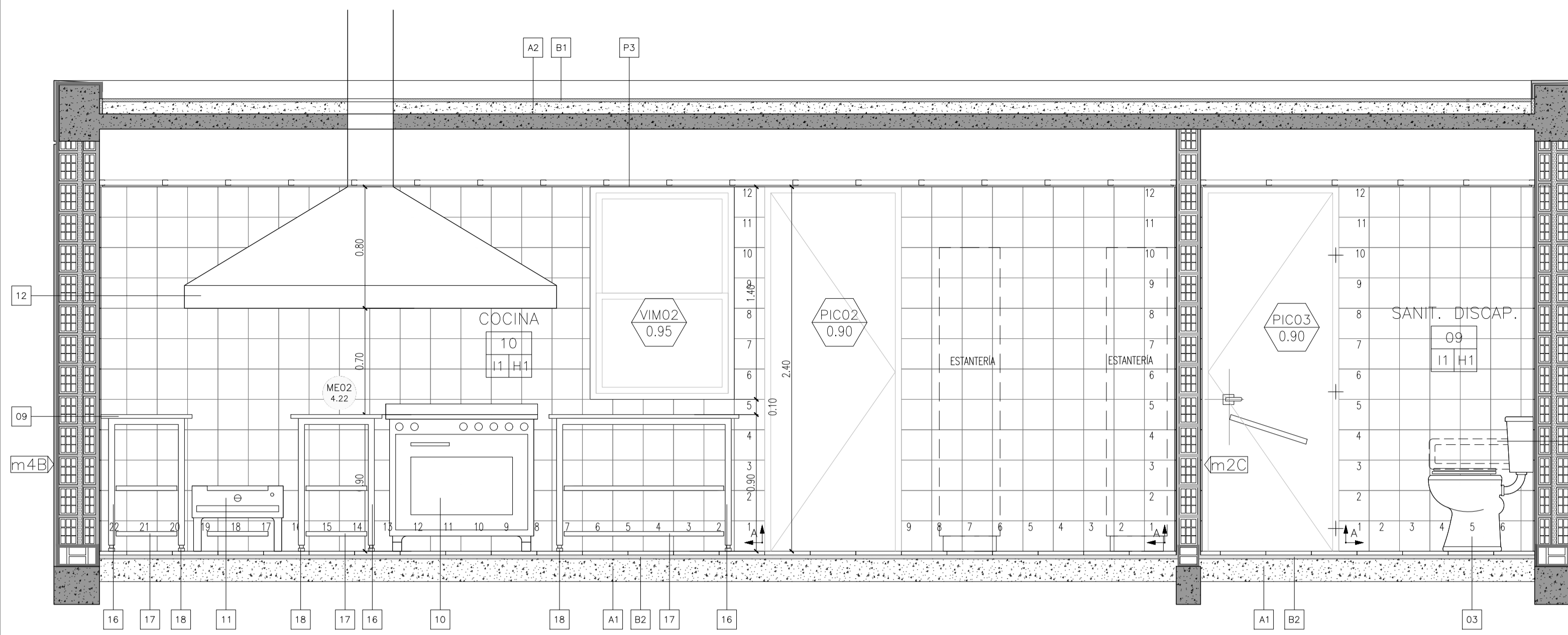
CORTE A-A
