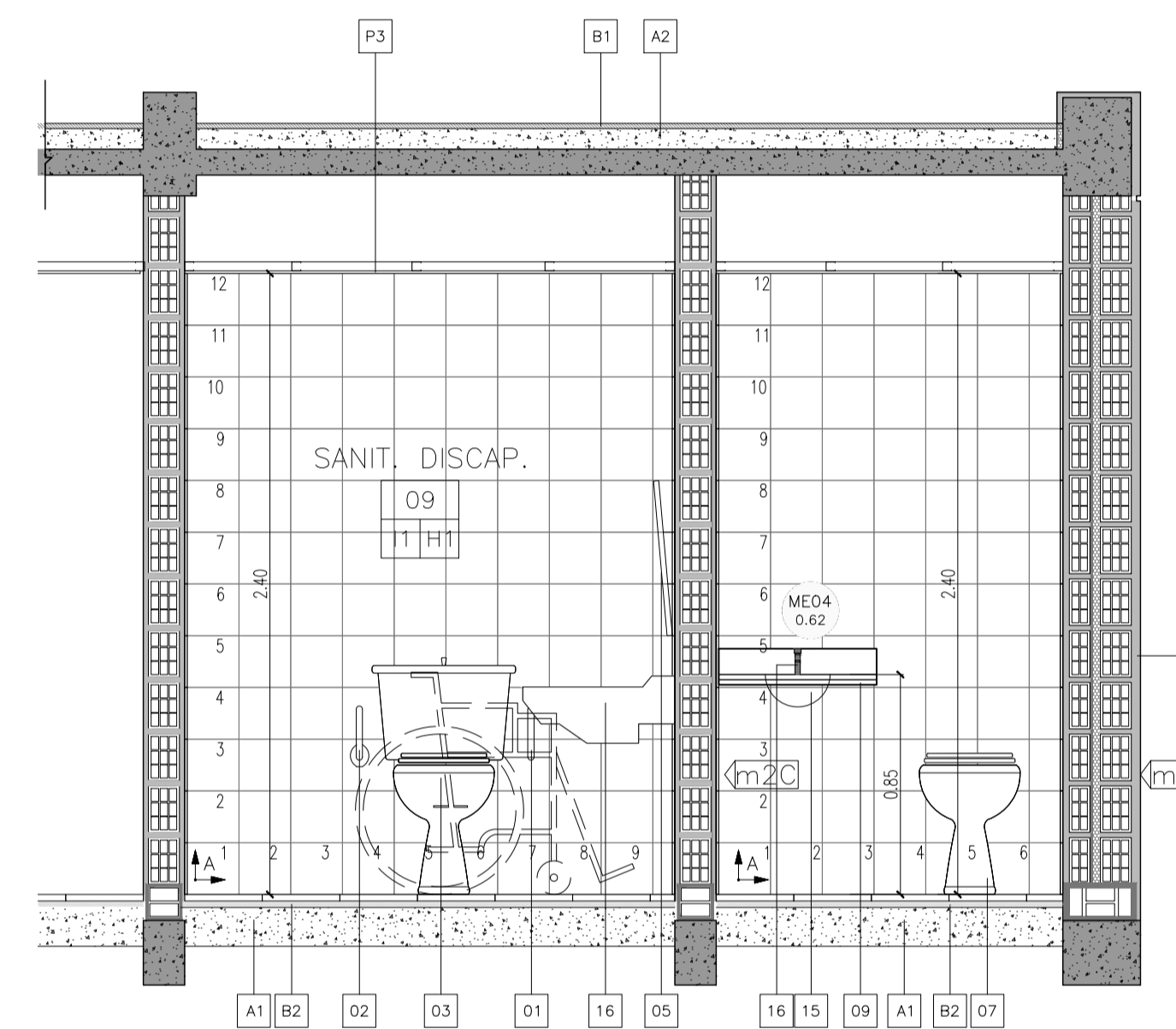
CORTE D-D
