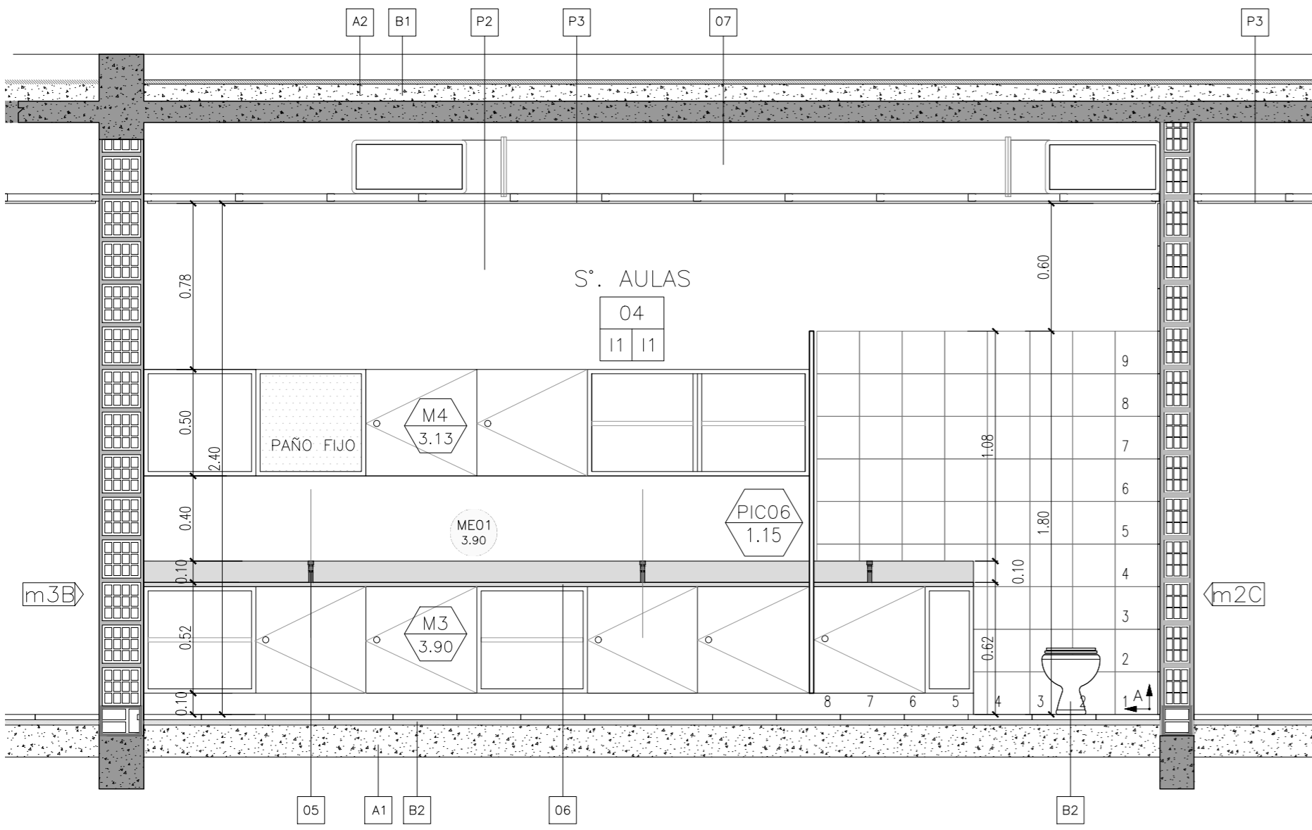
CORTE A-A
