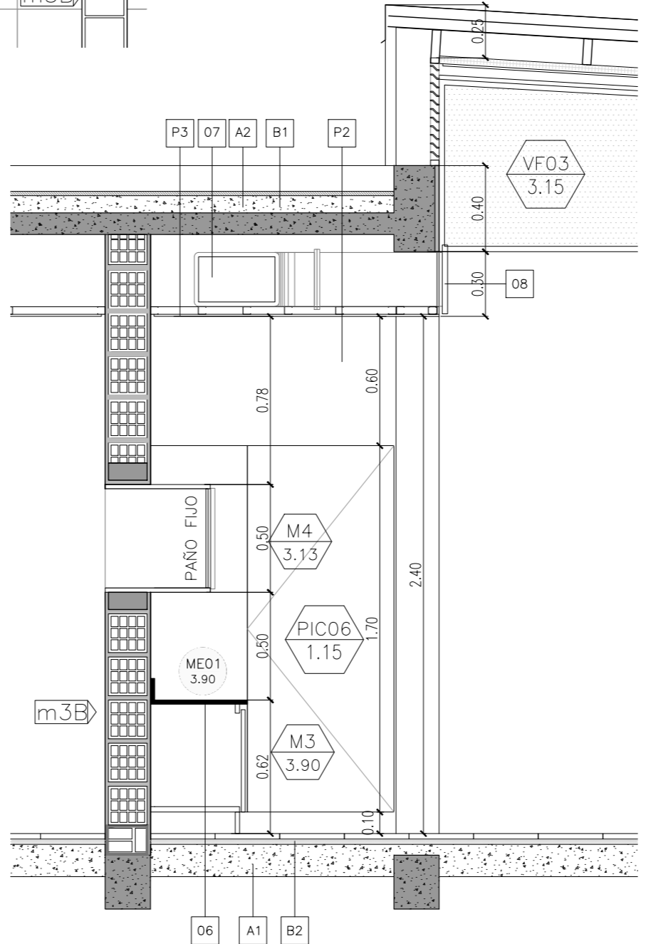
CORTE B-B
