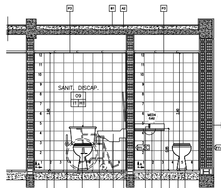
CORTE D-D
