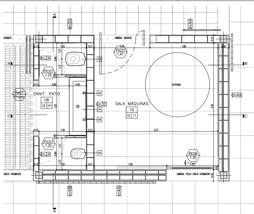
PLANTA
