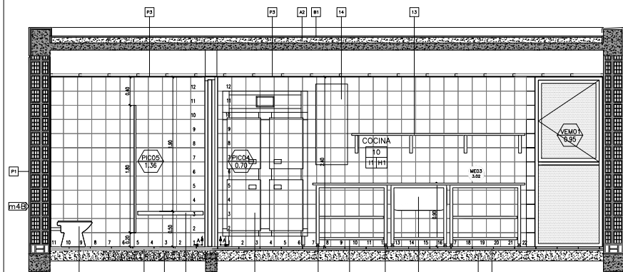
CORTE B-B
