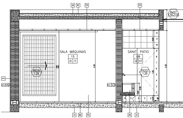
CORTE C-C
