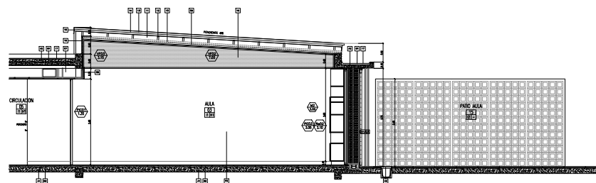
CORTE C-C
