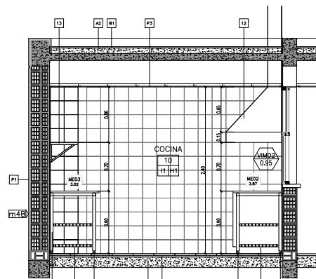
CORTE C-C
