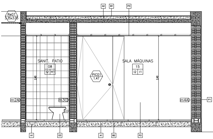
CORTE B-B
