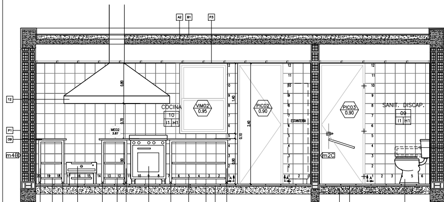
CORTE A-A
