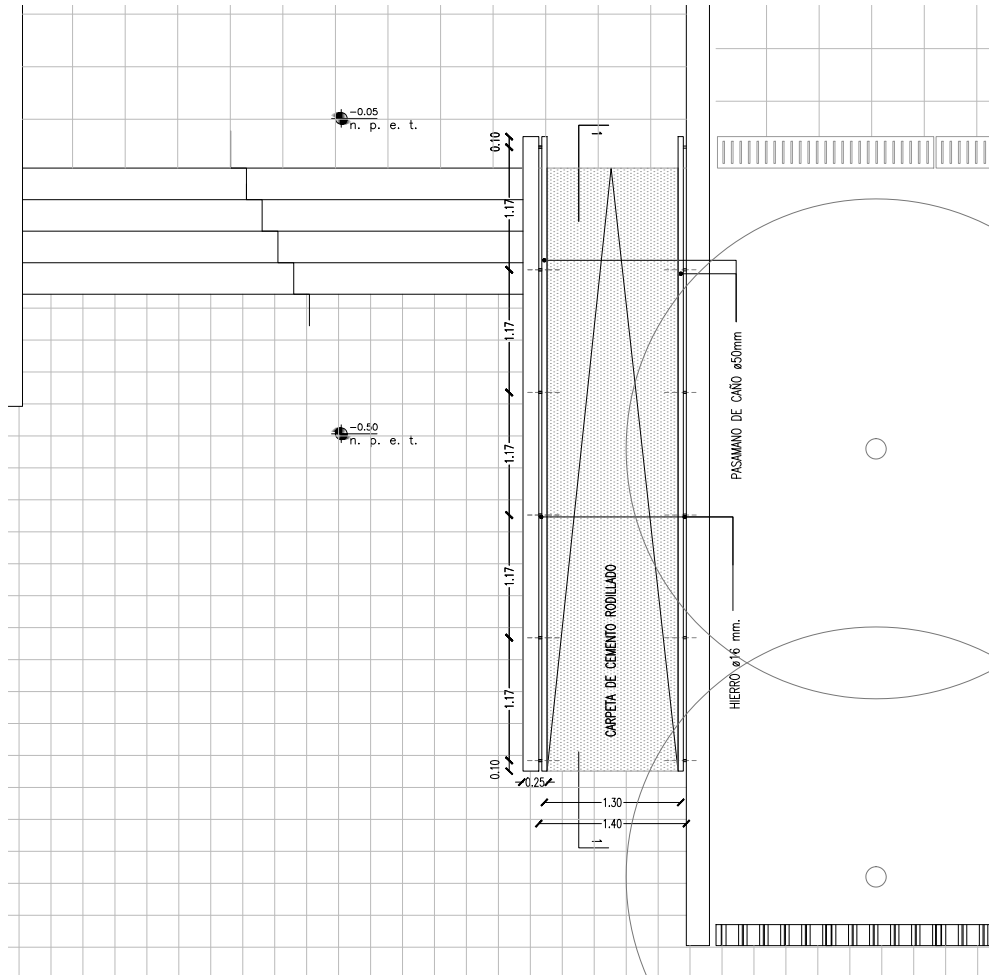
CORTE 1-1 ESC. 1:50
