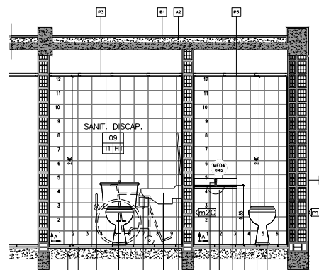
CORTE D-D
