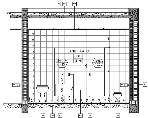
CORTE A-A
