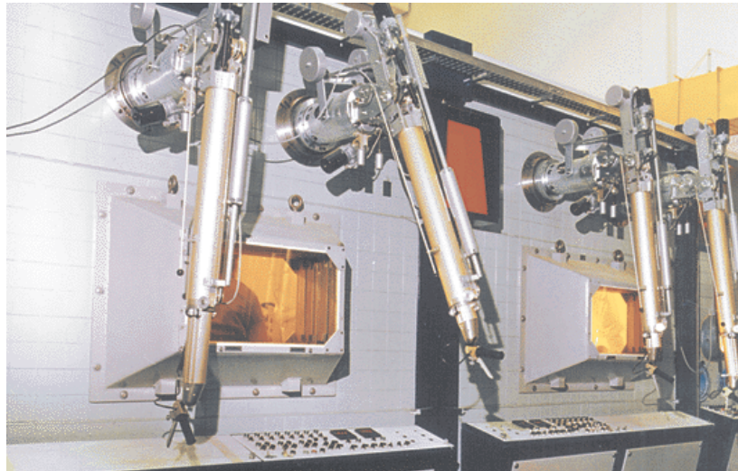
Celdas de procesos en la planta de producción de molibdeno 99 por fisión
