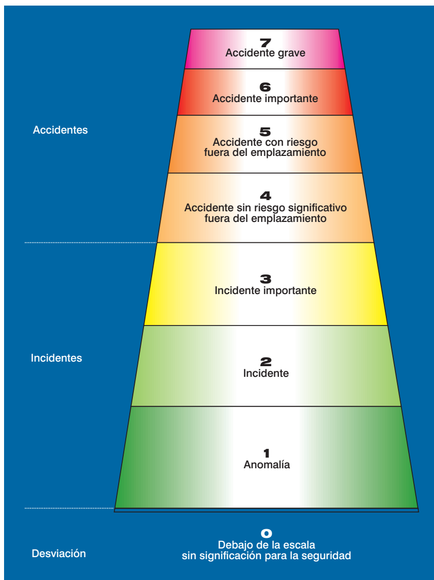
Figura 6. Escala Internacional de Sucesos Nucleares
