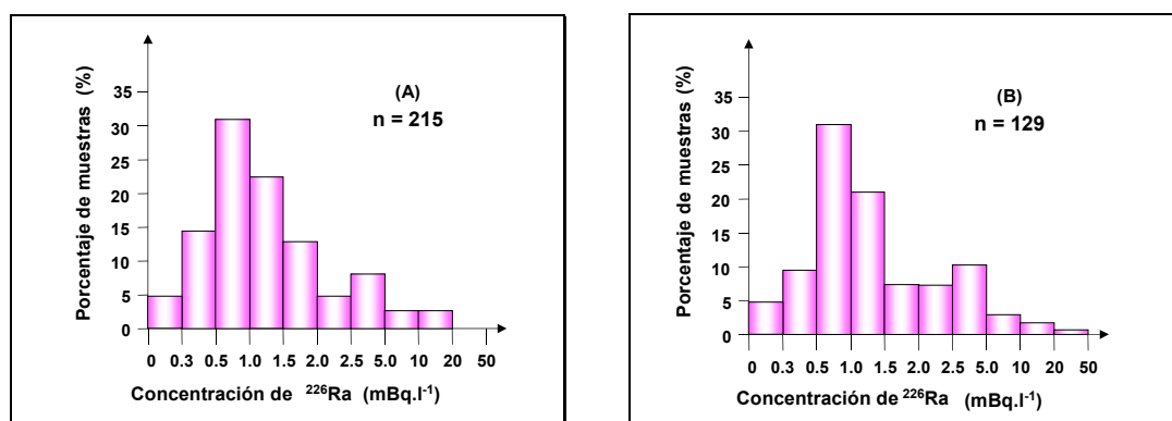
Figura 4. Distribución de frecuencias de concentración de ^{226}\text{Ra} en aguas potables de Argentina. Muestras provenientes de: (A) redes de distribución domiciliaria, (B) pozos privados.
