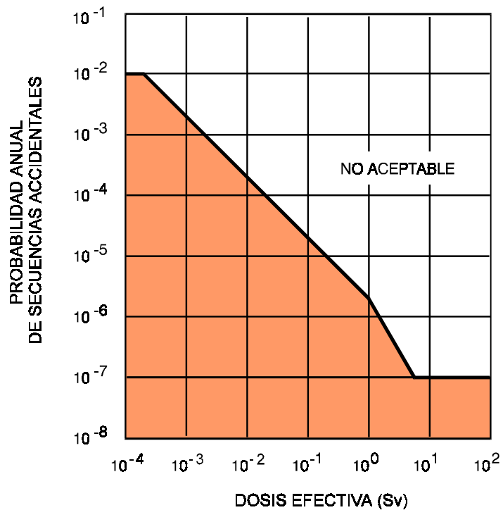
Figura 1 CURVA CRITERIO PARA EL PÚBLICO
