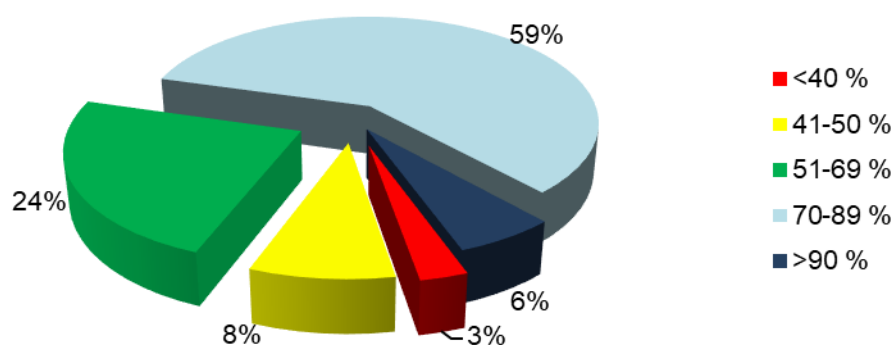
Figura 13. Horas totales mensuales expresadas como porcentaje de los diferentes rangos de humedad.
