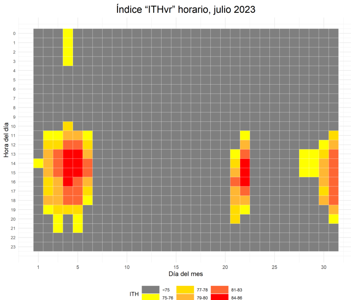
Figura 15. Distribución horaria diaria para cada valor del ITHvr calculado en base al registro de la estación automática para el mes de julio de 2023.
