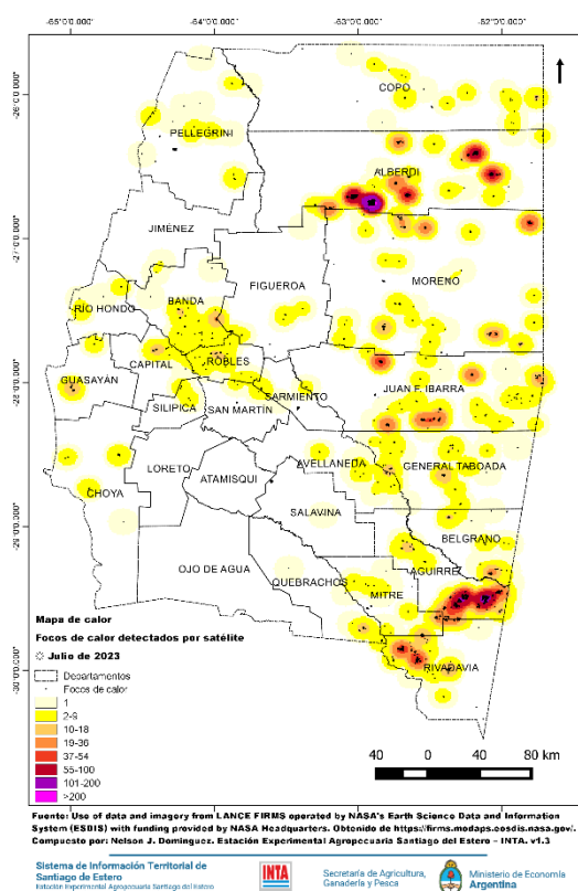
Figura 24. Focos de calor detectados por sensores satelitales y densidad de estos durante el mes de julio de 2023.
