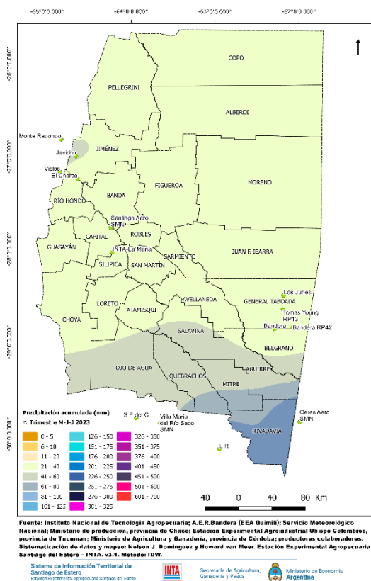
Figura 20. Precipitación acumulada (mm) entre mayo y julio de 2023.
