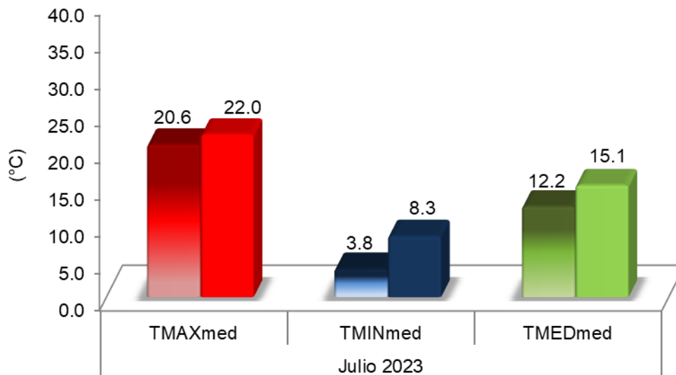
Figura 1. Valores medios mensuales de temperaturas máximas, mínimas y medias para el mes de julio. Referencias: colores degradados (julio serie 1991-2020), colores uniformes (julio 2023)
