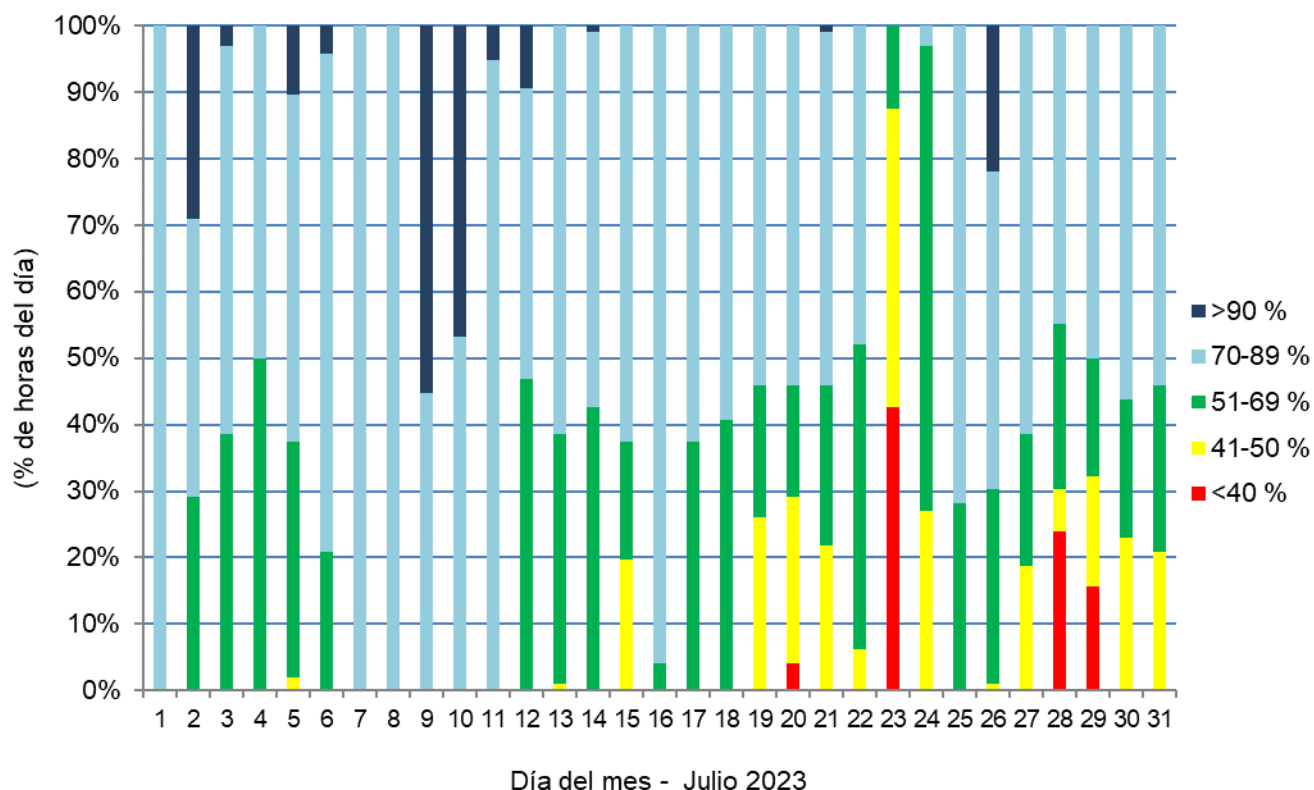
Figura 12. Duración horaria expresada como porcentaje del día para cada intervalo de humedad observado, en base al registro de la estación automática.
