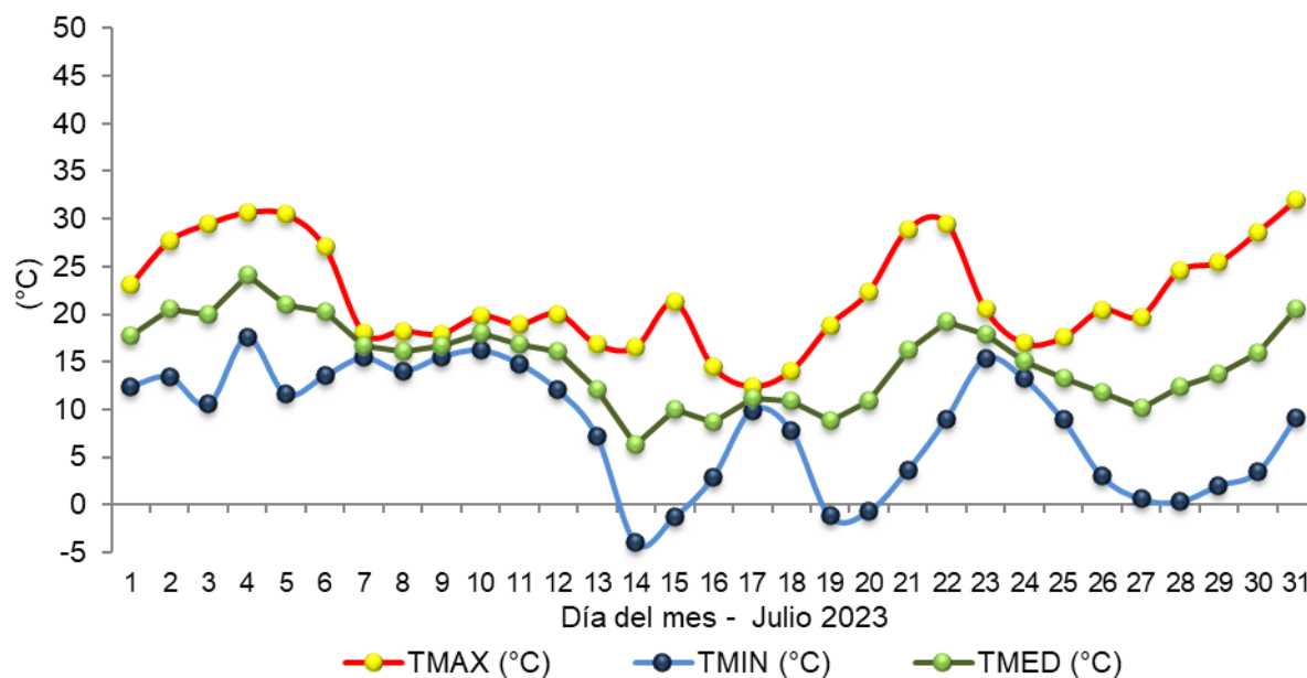
Figura 4. Valores diarios de temperatura para el mes de julio de 2023.
