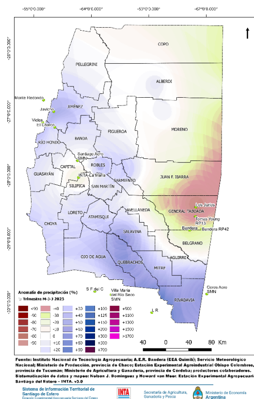
Figura 21. Anomalía de precipitación (%) entre mayo y julio de 2023.
