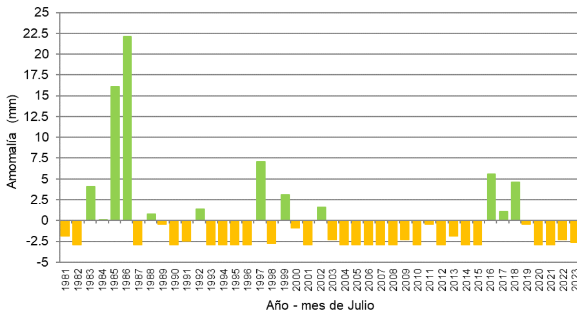
Figura 6. Anomalía de precipitación mensual (mm) para el mes de julio. Serie histórica (1981-2020).
