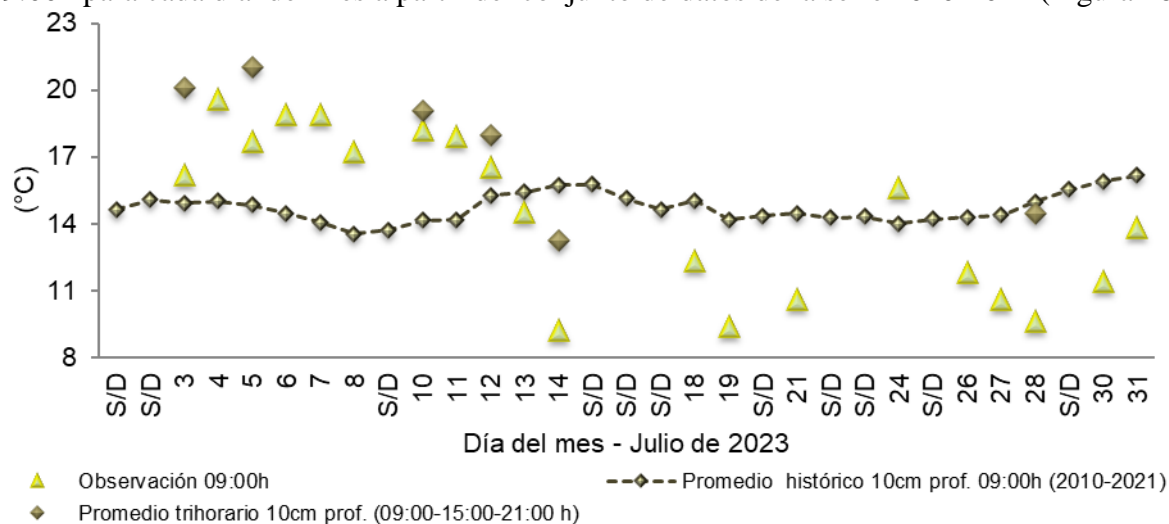
Figura 16. Valor de temperatura de suelo a las 09:00h suelo a 10cm bajo la superficie, valores medios trihorarios de temperatura de suelo a 10cm bajo la superficie. S/D: sin dato.
