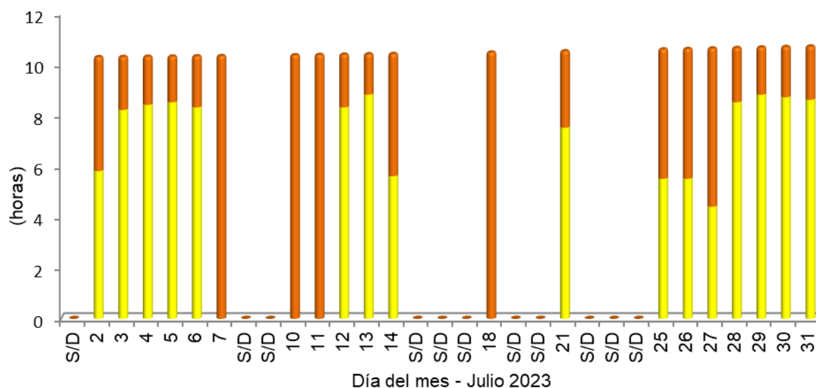
Figura 7. Valores de heliofanía efectiva con relación a la heliofanía teórica astronómica para cada día, expresados en horas y décimos de hora, registrados mediante un heliofanógrafo tipo Campbell-Stokes.
