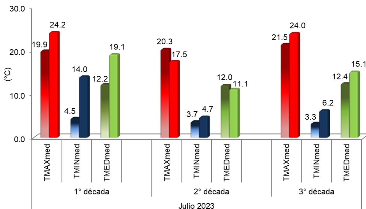
Figura 2. Valores medios de temperaturas máximas, mínimas y medias, agrupadas en períodos decadales, para el mes de julio. Referencias: colores degradados (julio serie 1991-2020), colores uniformes (julio 2023).
