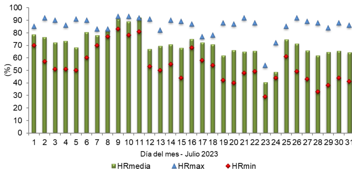
Figura 10. Valores diarios de humedad relativa (%).
