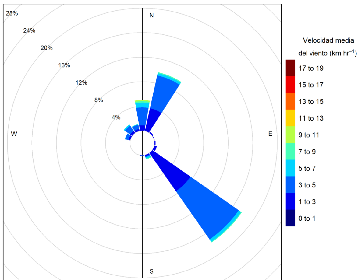
Figura 9. Porcentaje de la dirección del viento prevalente y porcentaje de cada intervalo de velocidad en cada una de las direcciones del viento para el mes de julio de 2023.
