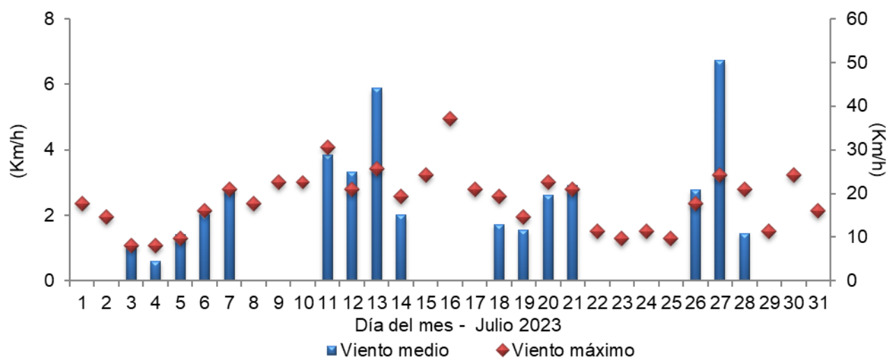
Figura 8. Valores de viento promedio diario a partir de anemómetro y, valor del viento máximo diario registrado por estación meteorológica automática.
