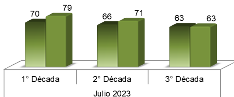
Figura 11. Valores medios de humedad relativa (%) agrupados por décadas para el mes de julio. Referencias: colores: degradados (julio serie 1989-2014), colores uniformes (julio 2022).
