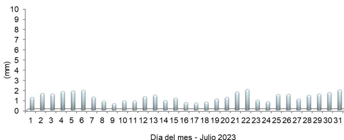
Figura 17. Valores diarios de evapotrasnpiración. Método Fao-Penman Monteith
