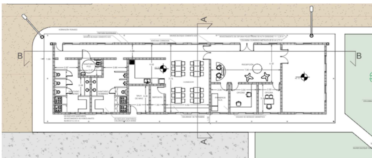
Plano CA Miramar "Oficina de administración y centro de interpretación con sala de primeros auxilios - Planta de arquitectura".
