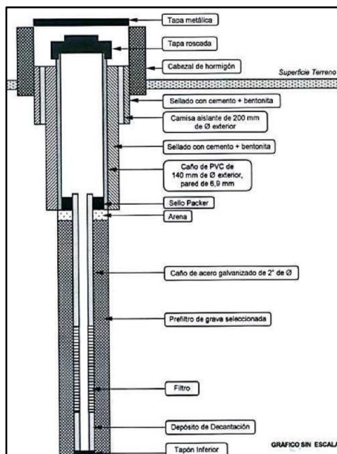
Figura 1. Esquema Pozo de Monitoreo
