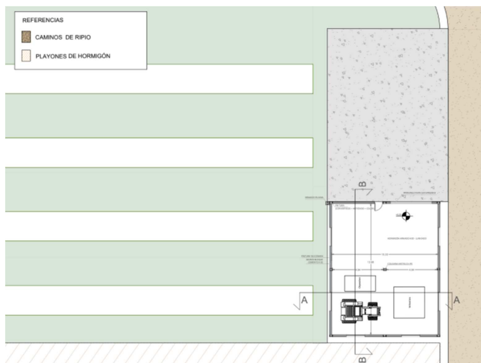
Plano CA Miramar "Sector de poda y compostaje"
