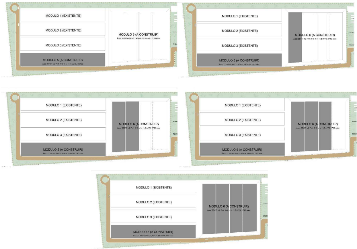
Esquema secuencia de llenado - Predio CA Miramar . Elaboración propia.
