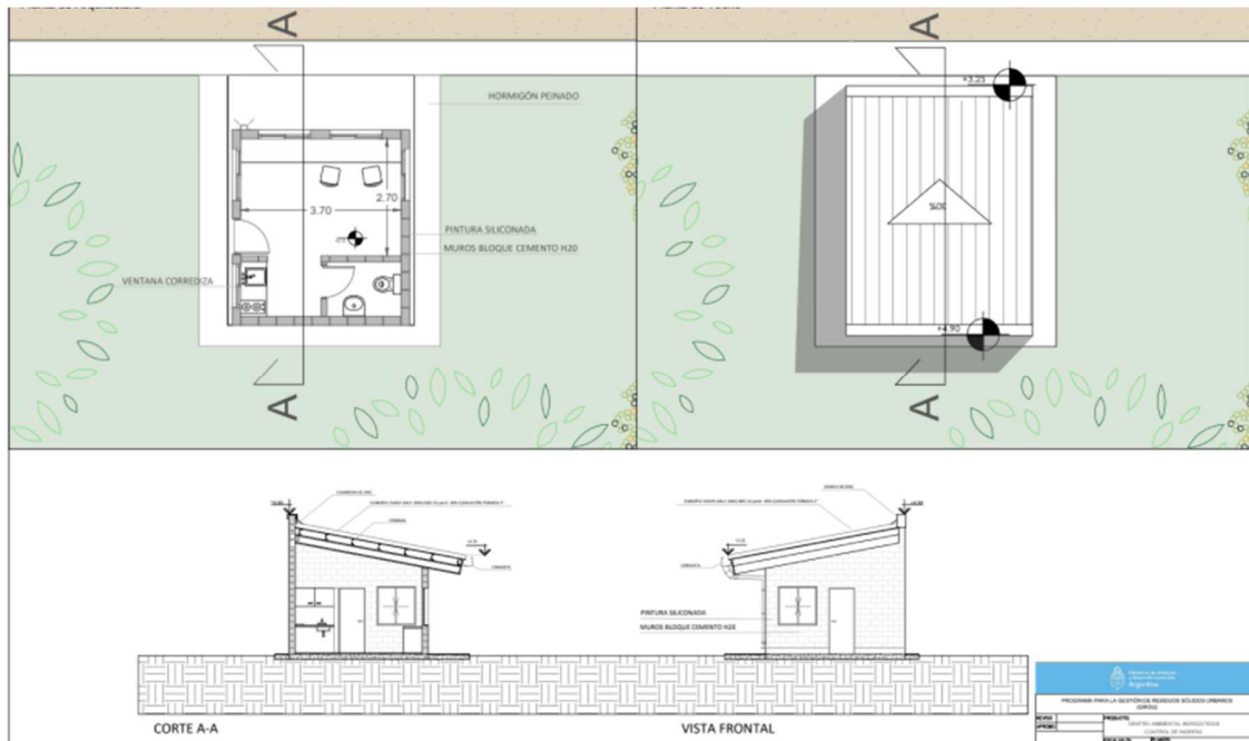
Plano CA Miramar “Control de ingreso y balanza”.
