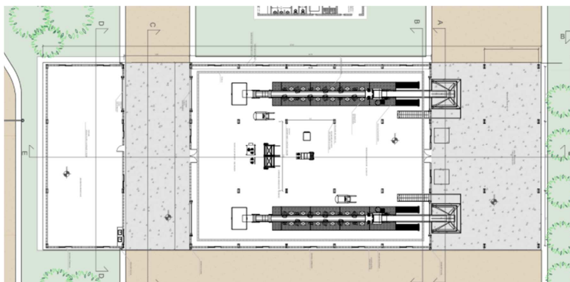
Plano CA Miramar "Planta de separación y clasificación"
