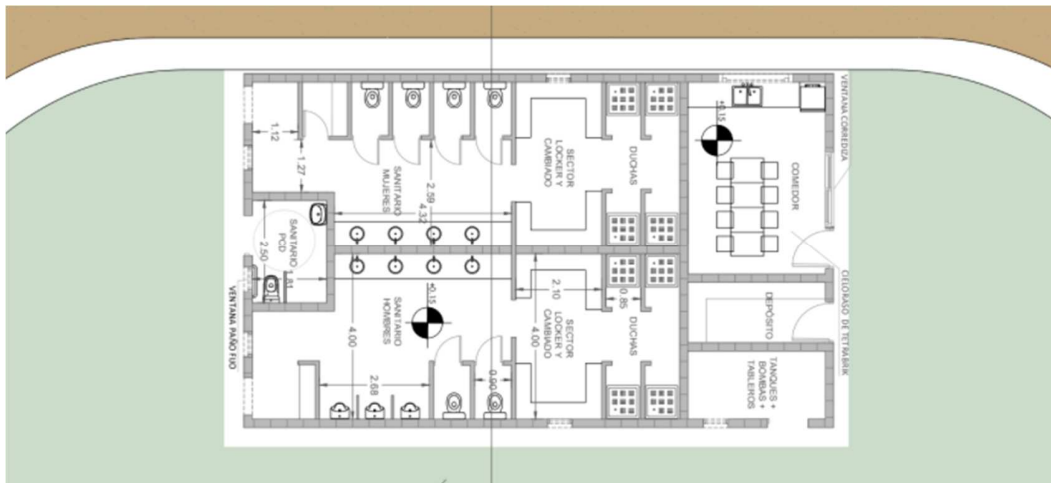
Plano CA Miramar "Vestuarios y sector de descanso"
