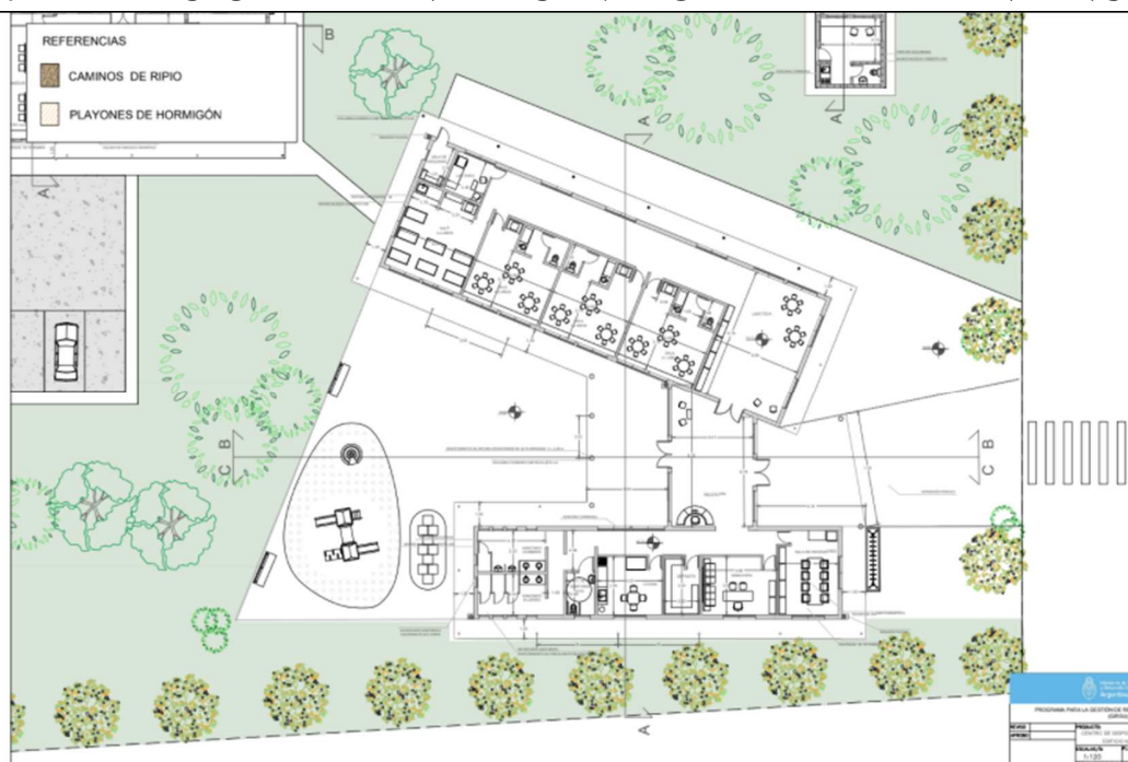
Plano CA Miramar "Centro de primera infancia"
